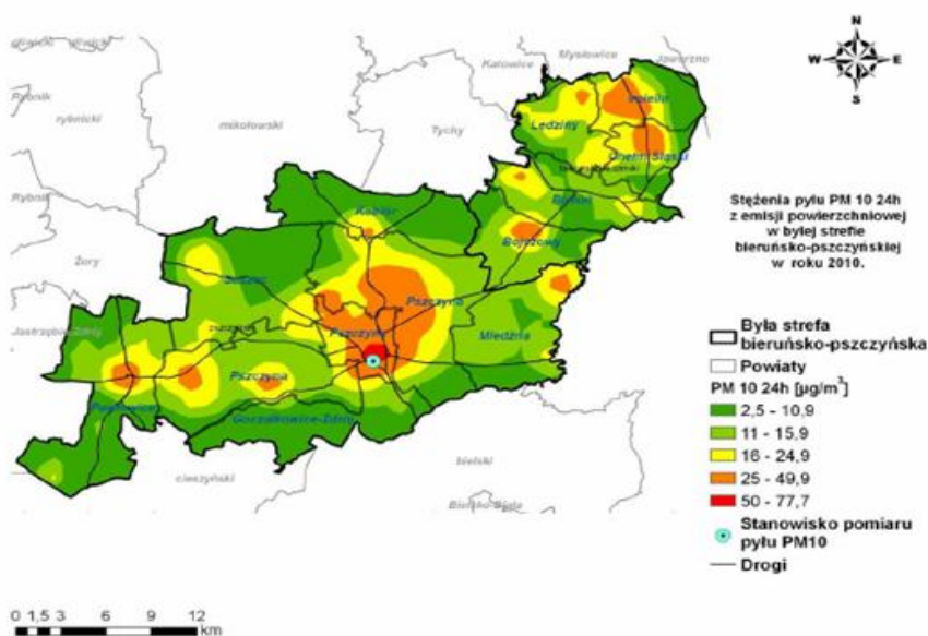
Rysunek 62. Stężenia pyłu zawieszonego PM 10 o okresie uśredniania wyników 24h w byłej strefie bieruńsko-pszczyńskiej pochodzące z emisji komunalnej w 2010 r.
