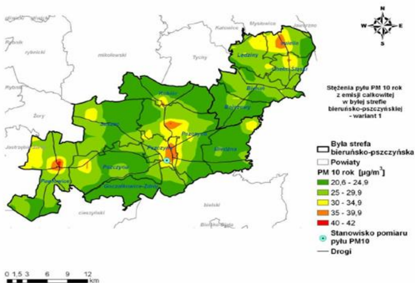
Rysunek 114. Stężenia pyłu zawieszonego PM10 o okresie uśredniania wyników rok pochodzące z emisji całkowitej w byłej strefie bieruńsko-pszczyńskiej po zastosowaniu wariantu 1
