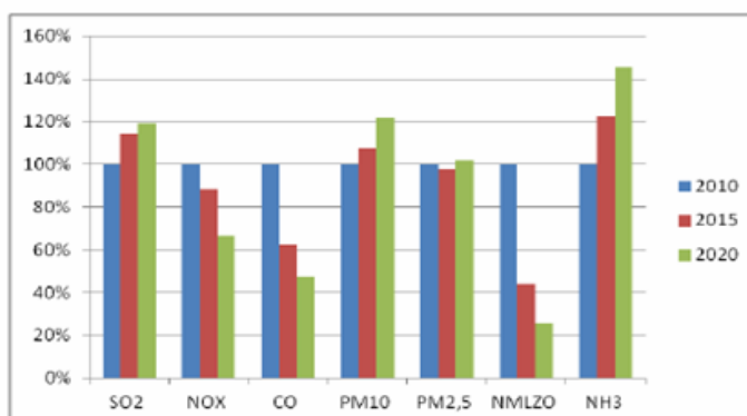
Rysunek 26. Prognoza emisji poszczególnych zanieczyszczeń pochodzących z komunikacji.
