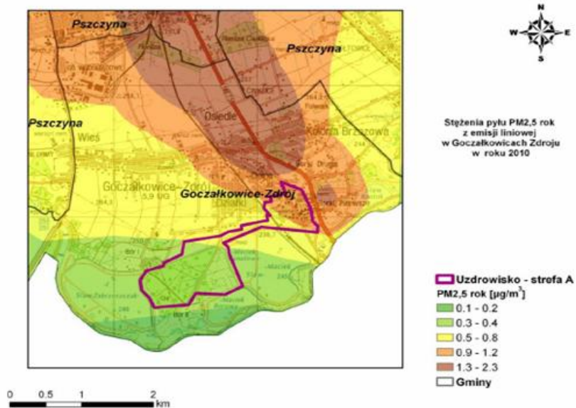
Rysunek 89. Stężenia pyłu zawieszonego PM 2,5 o okresie uśredniania wyników rok w Goczałkowicach – Zdroju pochodzące z emisji komunikacyjnej w 2010 r.
