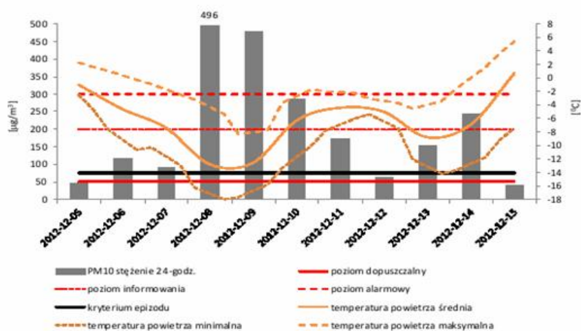
Rysunek 140. Średnie dobowe stężenie PM10 na tle wartości granicznych i temperatury powietrza od 5 do 15 grudnia 2012 roku dla Goczałkowic-Zdroju.
