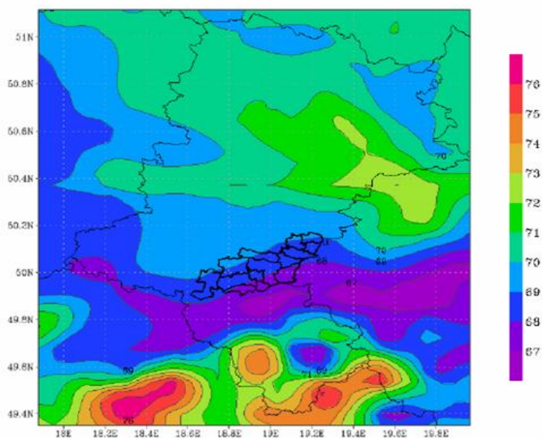
Rysunek 41. Rozkład średniej rocznej wartości wilgotności powietrza atmosferycznego w byłej strefie bieruńsko-pszczyńskiej w 2010 r.
