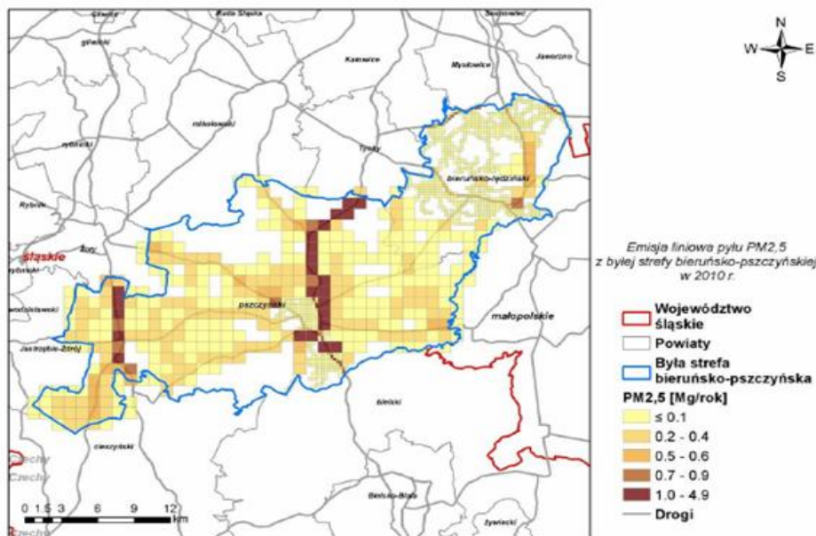
Rysunek 23. Emisja liniowa pyłu zawieszonego PM 2,5 w byłej strefie bieruńsko-pszczyńskiej w 2010 r.
