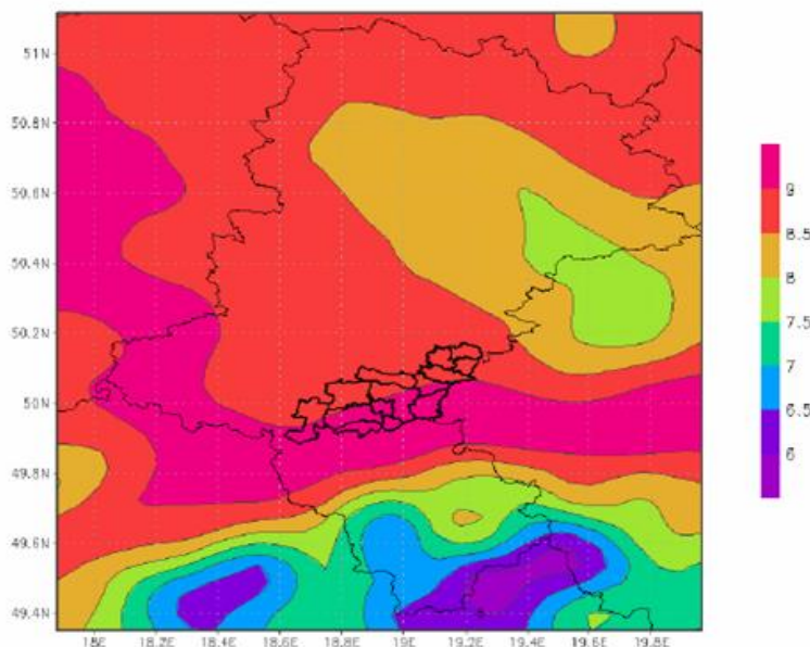
Rysunek 38. Rozkład średniej rocznej wartości temperatury powietrza w byłej strefie bieruńsko-pszczyńskiej w 2010 r.
