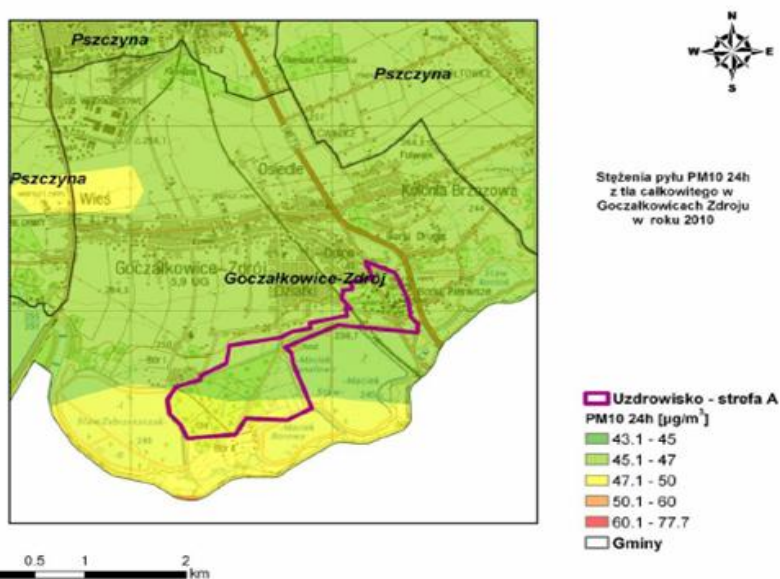
Rysunek 55. Stężenia PM 10 o okresie uśredniania wyników 24h w Goczałkowicach - Zdroju pochodzące z tła całkowitego w 2010 r.
