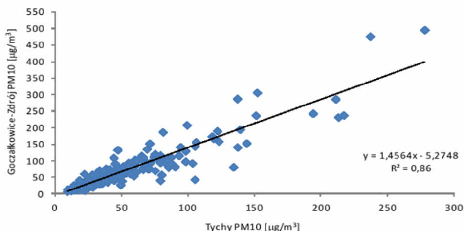
Rysunek 131. Zależność między stężeniem dobowym PM10 w Goczałkowicach-Zdroju a Tychami w okresie od 20 września 2012 r. do 19 września 2013 r.
