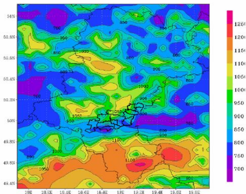
Rysunek 42. Rozkład średniej miesięcznej wartości miąższości mieszania w strefie bieruńsko-pszczyńskiej w roku 2010.
