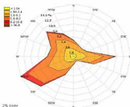
Rysunek 34. Róża wiatrów dla byłej strefy bieruńsko-pszczyńskiej – sezon letni w 2010 r.
