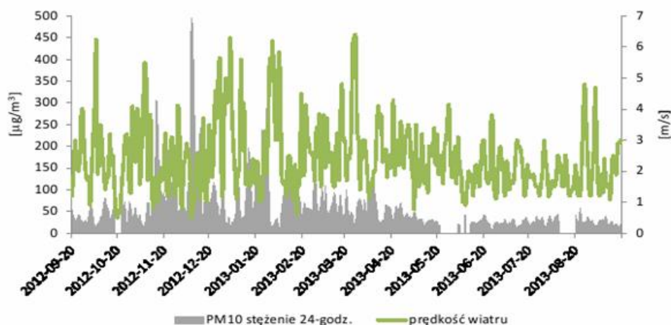
Rysunek 135. Średnie dobowe stężenie PM10 na tle średniej dobowej prędkości wiatru na stacji Katowice-Muchowiec od 20 września 2012 r. do 19 września 2013 r. dla Goczałkowic-Zdroju.
