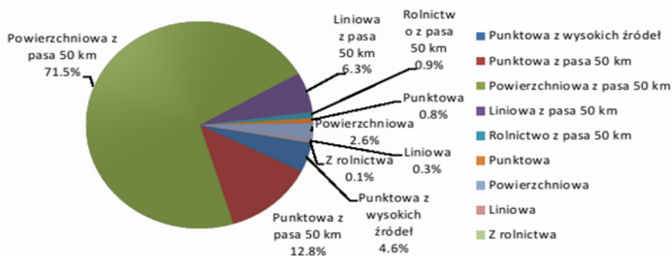
Rysunek 31. Procentowy udział typów źródeł w bilansie emisji pyłu PM2,5 dla byłej strefy bieruńsko-pszczyńskiej w 2010 r.
