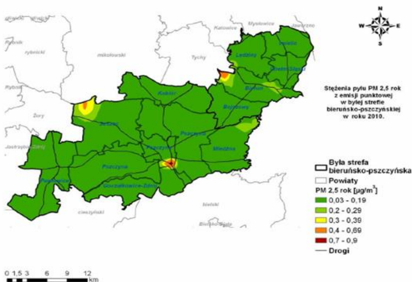
Rysunek 84. Stężenia pyłu zawieszonego PM 2,5 o okresie uśredniania wyników rok w byłej strefie bieruńsko-pszczyńskiej pochodzące z emisji punktowej w 2010 r.
