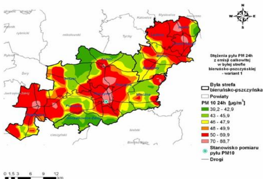
Rysunek 113. Stężenia pyłu zawieszonego PM 10 o okresie uśredniania wyników 24h pochodzące z emisji całkowitej w byłej strefie bieruńsko-pszczyńskiej po zastosowaniu wariantu 1
