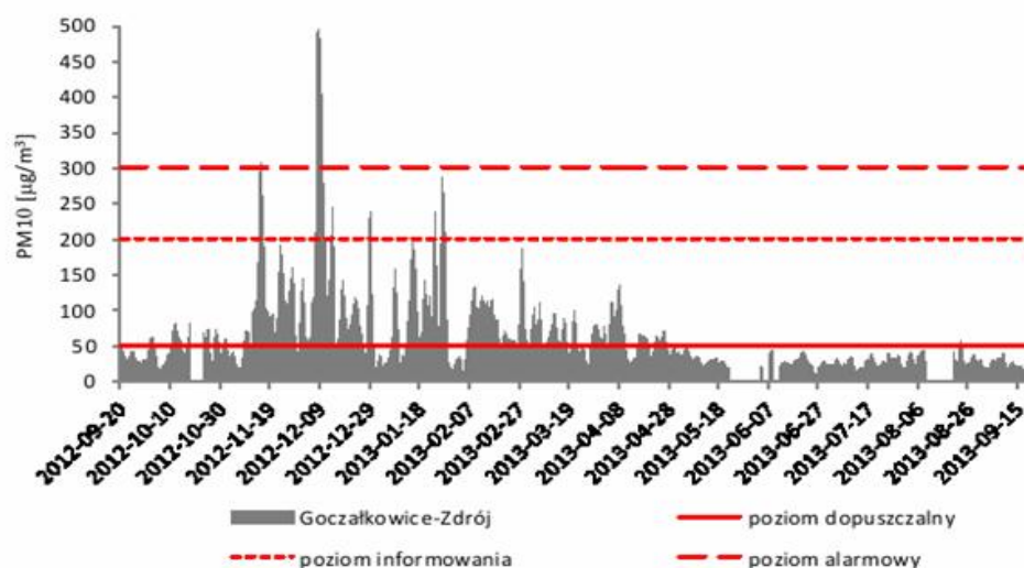
Rysunek 129. Stężenie średnie dobowe PM10 w okresie od 20.09.2012 r. do 19.09.2013 r. na tle poziomu dopuszczalnego, poziomu informowania i alarmowego dla Goczałkowic-Zdroju.
