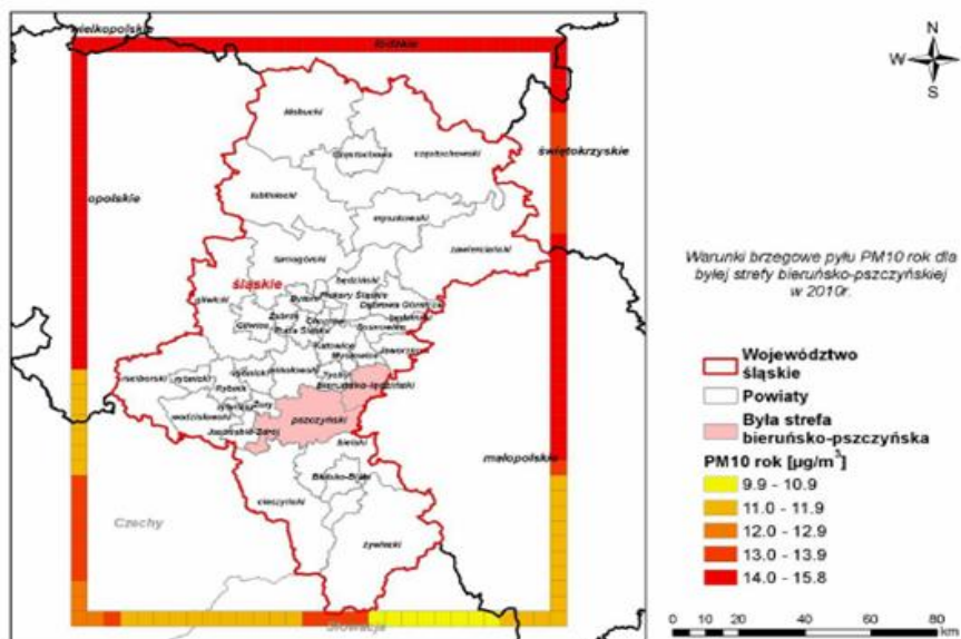
Rysunek 10. Warunki brzegowe pyłu zawieszonego PM10 dla byłej strefy bieruńsko-pszczyńskiej w 2010r.
