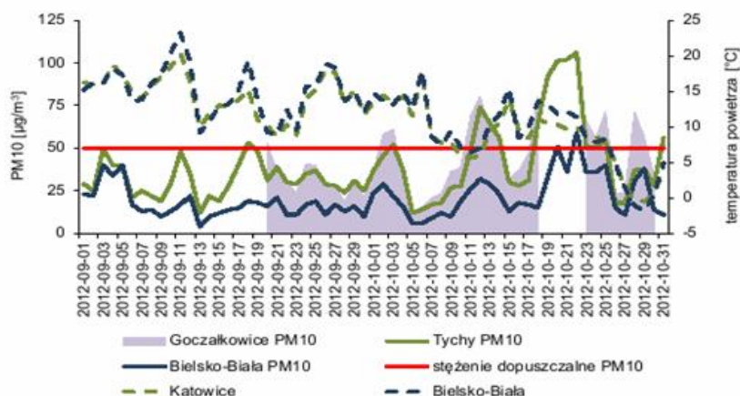
Rysunek 125. Średnie dobowe stężenie PM10 na stacji Tychy i Bielsko-Biala na tle średniej dobowej temperatury powietrza na stacji Katowice i Bielsko-Biala
