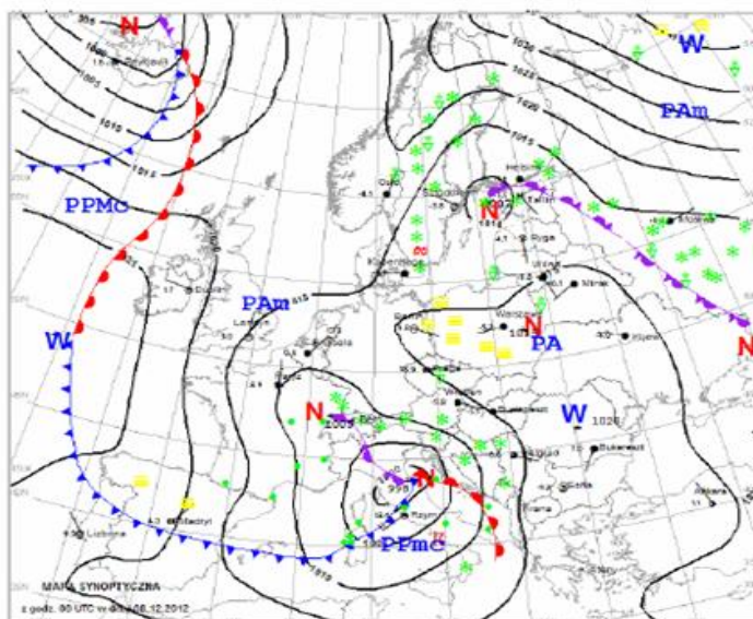
Rysunek 139. Mapa synoptyczna z godz. 0 UTC w dniu 8 grudnia 2012 r.
