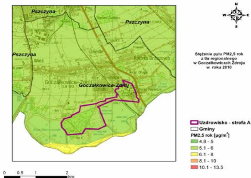
Rysunek 81. Stężenia PM 2,5 o okresie uśredniania wyników rok w Goczałkowicach - Zdroju pochodzące z tła regionalnego w 2010 r.
