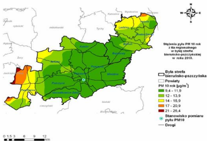
Rysunek 52. Stężenia PM10 o okresie uśredniania wyników rok w byłej strefie bieruńsko-pszczyńskiej pochodzące z tła regionalnego w 2010 r.
