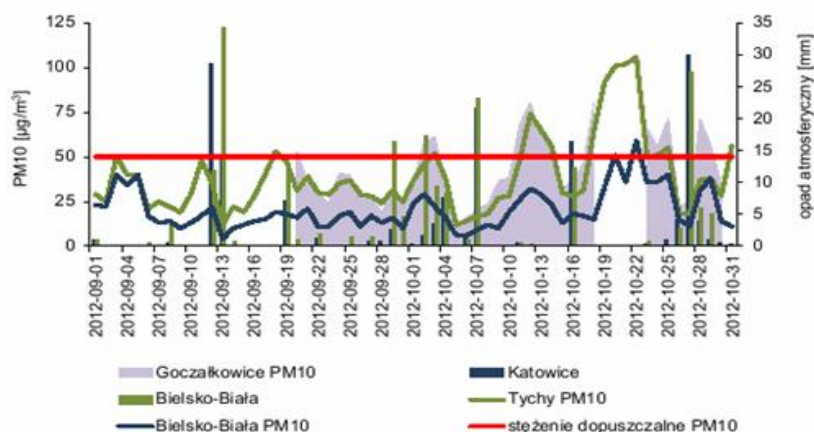
Rysunek 127. Średnie dobowe stężenie PM10 na stacji Tychy i Bielsko-Biała na tle sumy dobowej opadu atmosferycznego na stacji Katowice i Bielsko-Biała
