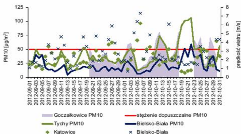
Rysunek 128. Średnie dobowe stężenie PM10 na stacji Tychy i Bielsko-Biała na tle średniej dobowej prędkości wiatru na stacji Katowice i Bielsko-Biała
