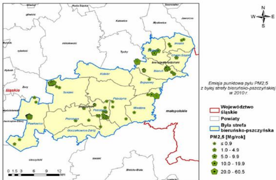
Rysunek 21. Emisja pyłu zawieszonego PM 2,5 ze źródeł punktowych w byłej strefie bieruńsko-pszczyńskiej w 2010 r.
