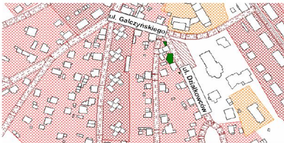
Rysunek 62. Mapa przekroczeń wskaźnika LDWN. Rejon parkingu przy ul. Działkowców.
