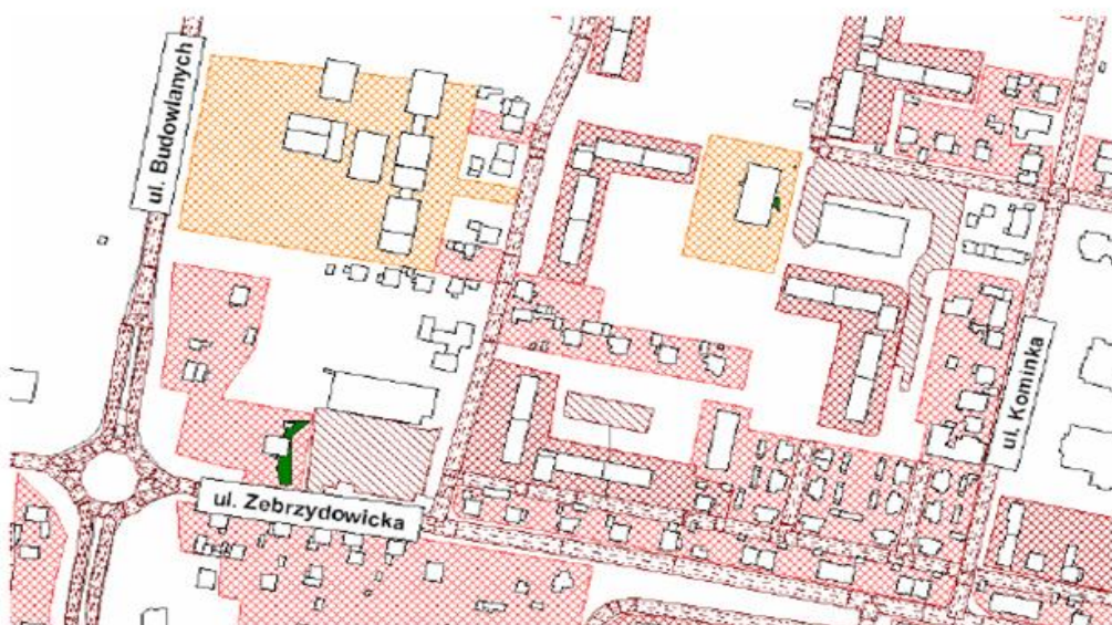
Rysunek 68. Mapa przekroczeń wskaźnika LDWN. Rejon przy ulic Zebrzydowickiej i Kominka
