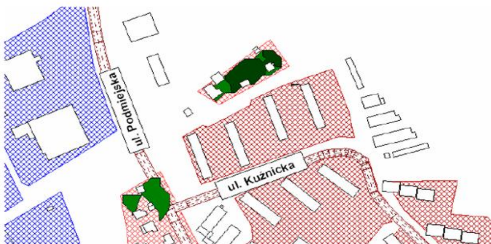
Rysunek 66. Mapa przekroczeń wskaźnika LDWN. Rejon ul. Kuźnickiej.
