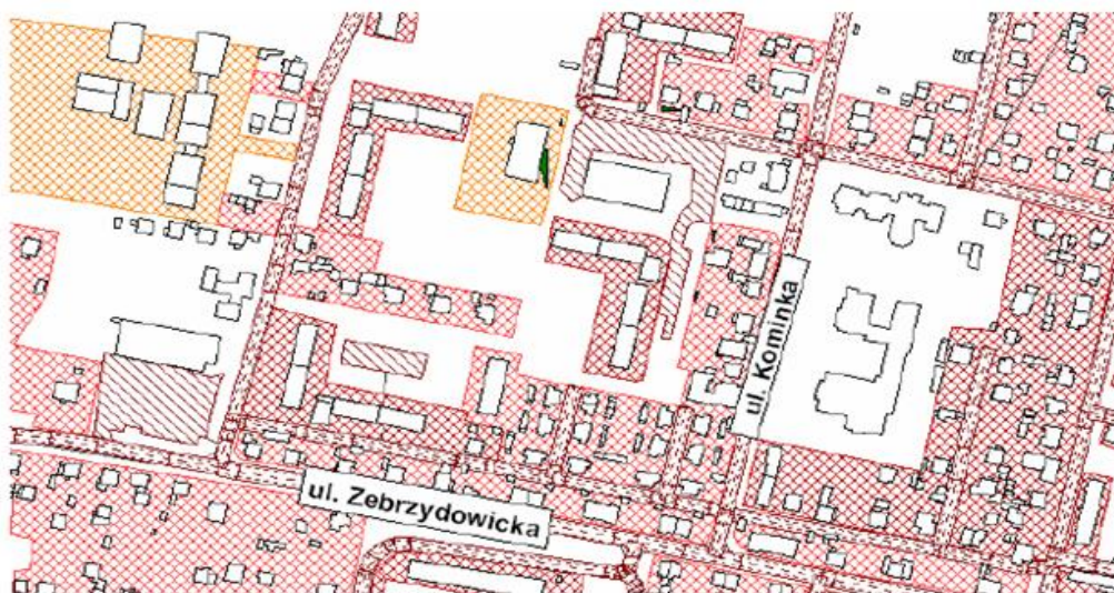
Rysunek 93. Mapa przekroczeń wskaźnika LN. Rejon przy ul. Zebrzydowskiej i Kominka
