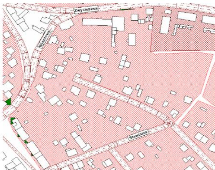
Rysunek 5. Zaktualizowana mapa przekroczeń (dla wartości dopuszczalnych z 2012 r.). Rejon ulic Zwycięstwa i Wjazdowej [2].
