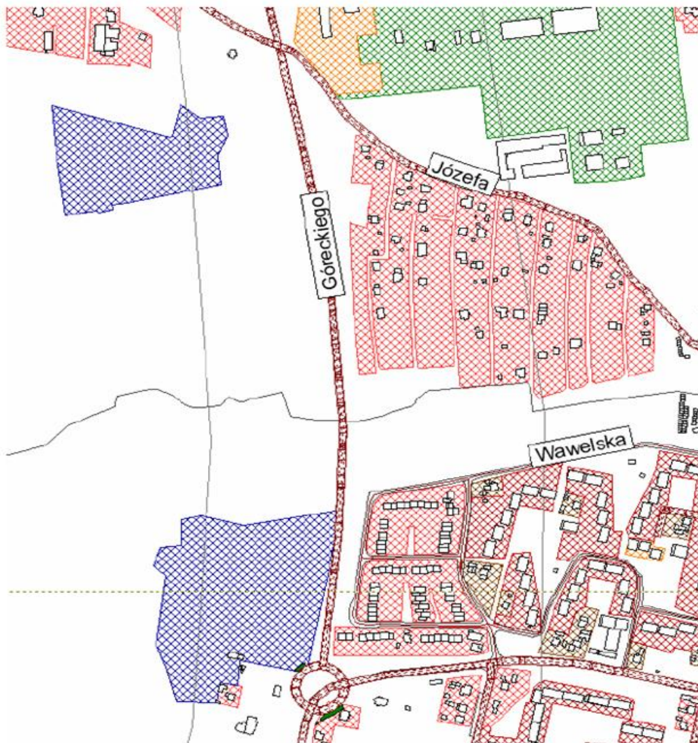
Rysunek 35. Mapy przekroczeń dla ul. Góreckiego, od ul. Budowlanych do ul. Józefa w Rybniku – mapy przekroczeń dla wartości LN [1]
