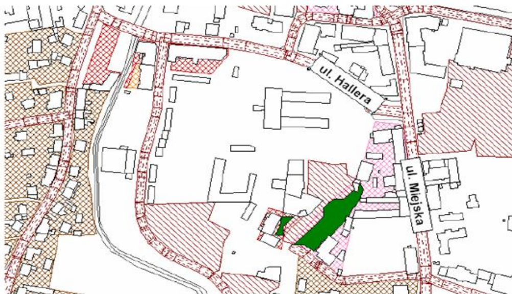
Rysunek 99. Mapa przekroczeń wskaźnika LN. Rejon przy ul. Miejskiej.
