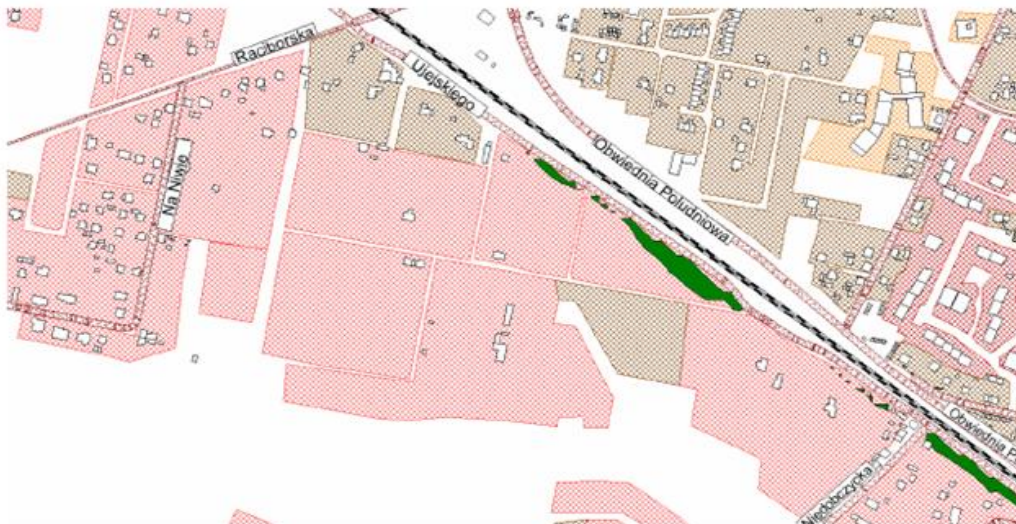
Rysunek 52. Zaktualizowana mapa przekroczeń (dla wartości dopuszczalnych z 2012 r.). Rejon od ul. Raciborskiej do ul. Niedobczyckiej [2].
