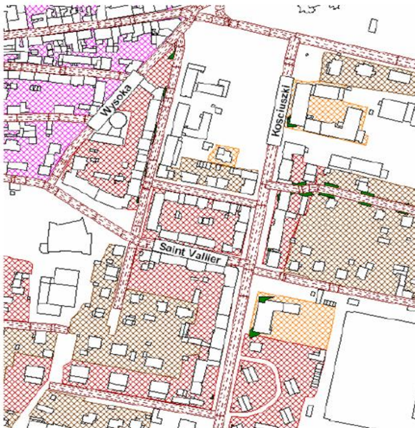
Rysunek 14. Zaktualizowana mapa przekroczeń (dla wartości dopuszczalnych z 2012 r.). Rejon wzdłuż ulic Kościuszki, Wysokiej i Saint Vallier [2].
