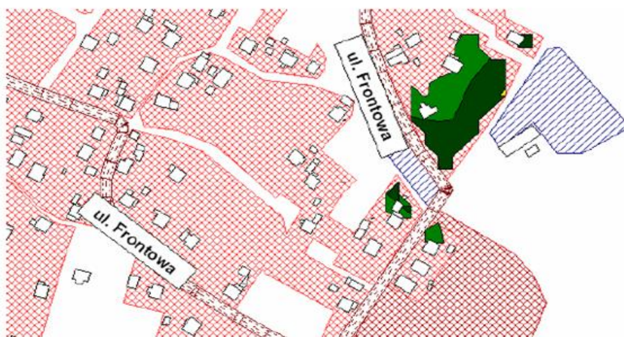
Rysunek 82. Mapa przekroczeń wskaźnika LDWN. Rejon przy ul. Frontowej
