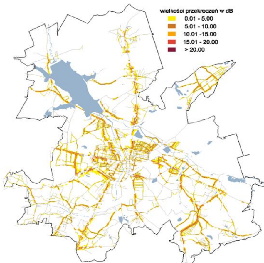
Rysunek 14. Tereny zagrożone hałasem drogowym (wskaźnik L_{DWN} ) [2].
