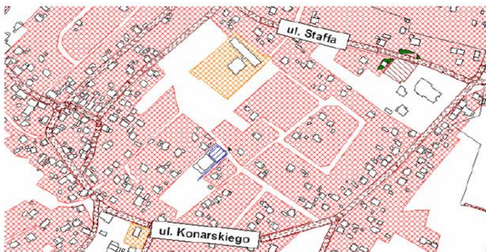
Rysunek 76. Mapa przekroczeń wskaźnika LDWN. Rejon przy ul. Konarskiego i Staffa.
