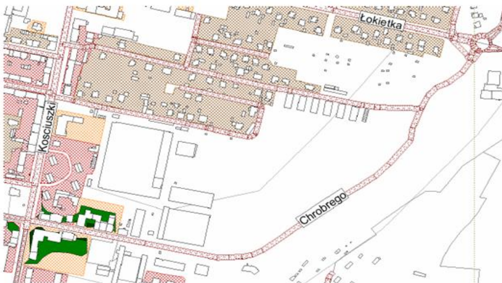
Rysunek 17. Mapy przekroczeń dla ul. Chrobrego, od ul. Kościuszki do ul. Łokietka w Rybniku – mapy przekroczeń dla wartości LDWN [1]
