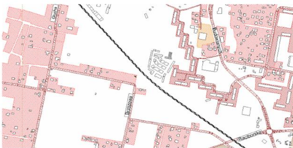
Rysunek 47. Zaktualizowana mapa przekroczeń (dla wartości dopuszczalnych z 2012 r.). Rejon od ul. Głuchej do ul. Raciborskiej [2].
