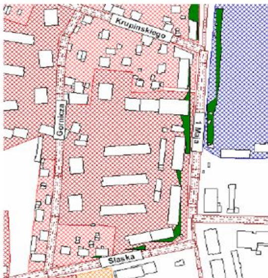
Rysunek 22. Zaktualizowana mapa przekroczeń (dla wartości dopuszczalnych z 2012 r.). Rejon ulic 1 Maja i Śląskiej [2].
