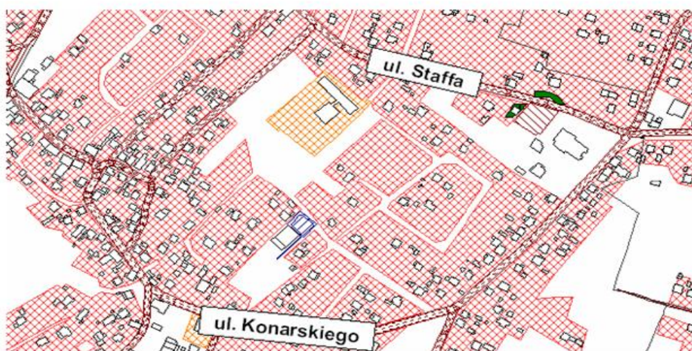
Rysunek 97. Mapa przekroczeń wskaźnika LN. Rejon przy ul. Konarskiego i Staffa.
