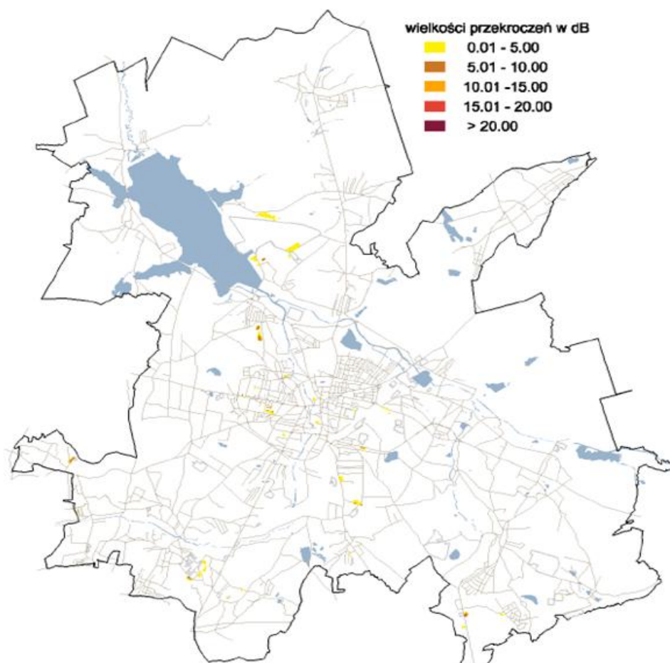
Rysunek 16. Tereny zagrożone hałasem przemysłowym (wskaźnik L_{DWN} ) [12].
