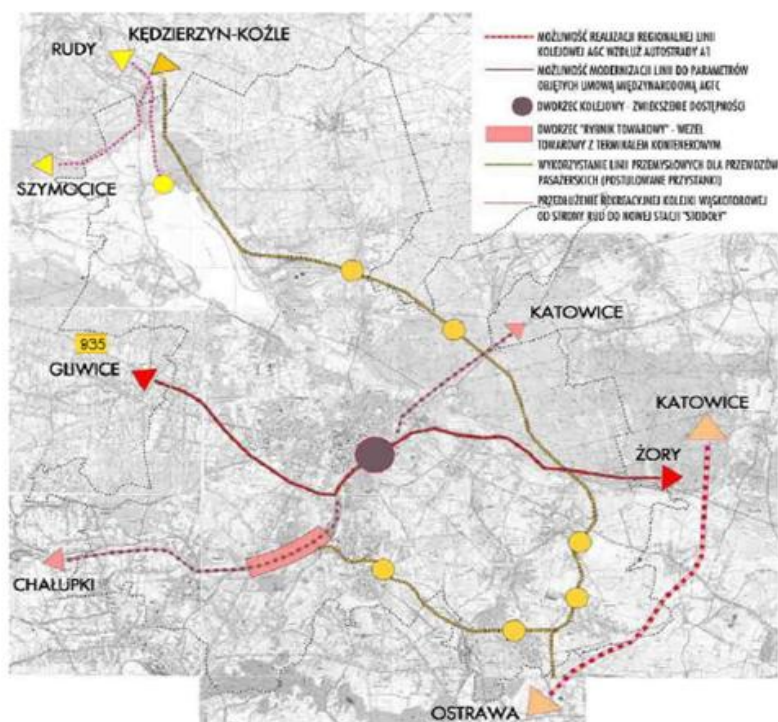
Rysunek 10. Komunikacja kolejowa w Mieście Rybnik [3].
