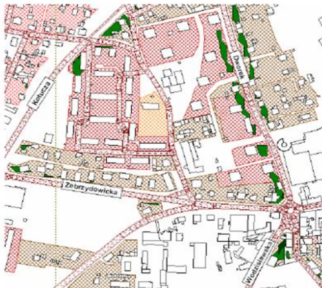
Rysunek 30. Zaktualizowana mapa przekroczeń (dla wartości dopuszczalnych z 2012 r.). Rejon wzdłuż ulic Kotucza i Dworek [2].
