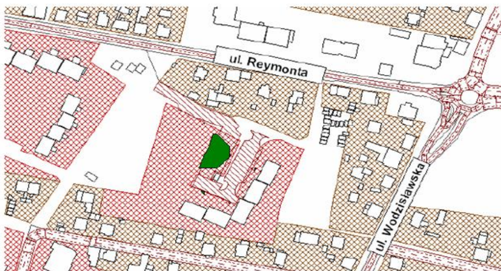
Rysunek 100. Mapa przekroczeń wskaźnika L. Rejon przy ul. Reymonta.
