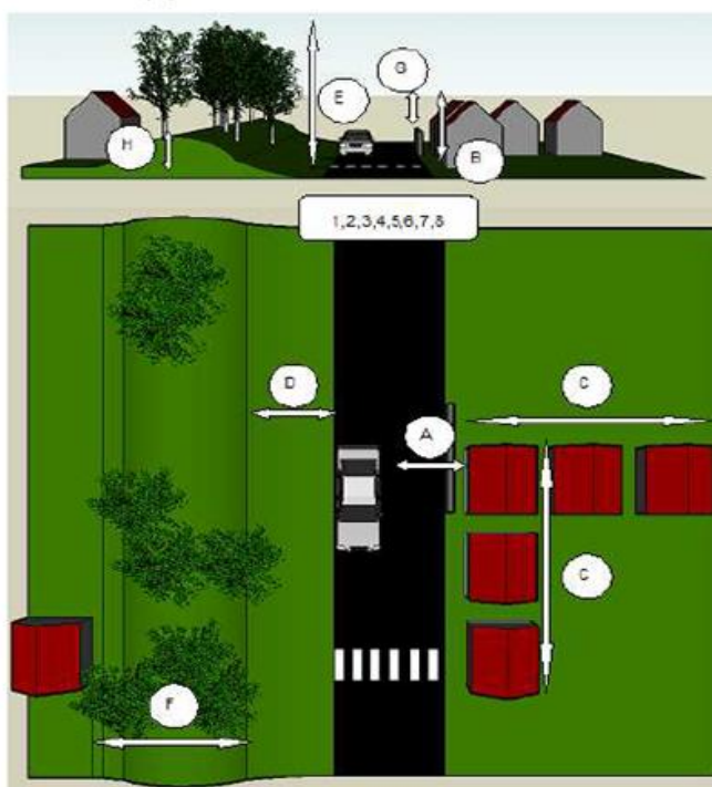
Rysunek 17. Wielkości wpływające na emisję i rozchodzenie się hałasu – hałas drogowy [2].
