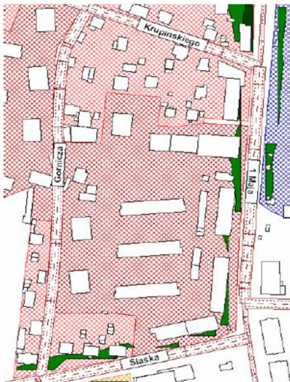
Rysunek 4. Zaktualizowana mapa przekroczeń (dla wartości dopuszczalnych z 2012 r.). Rejon ulic 1 Maja i Śląskiej [2].
