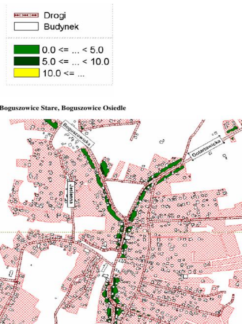
Rysunek 1. Zaktualizowana mapa przekroczeń (dla wartości dopuszczalnych z 2012 r.). Rejon skrzyżowania ulic Boguszowickiej i Gotartowickiej [2].
