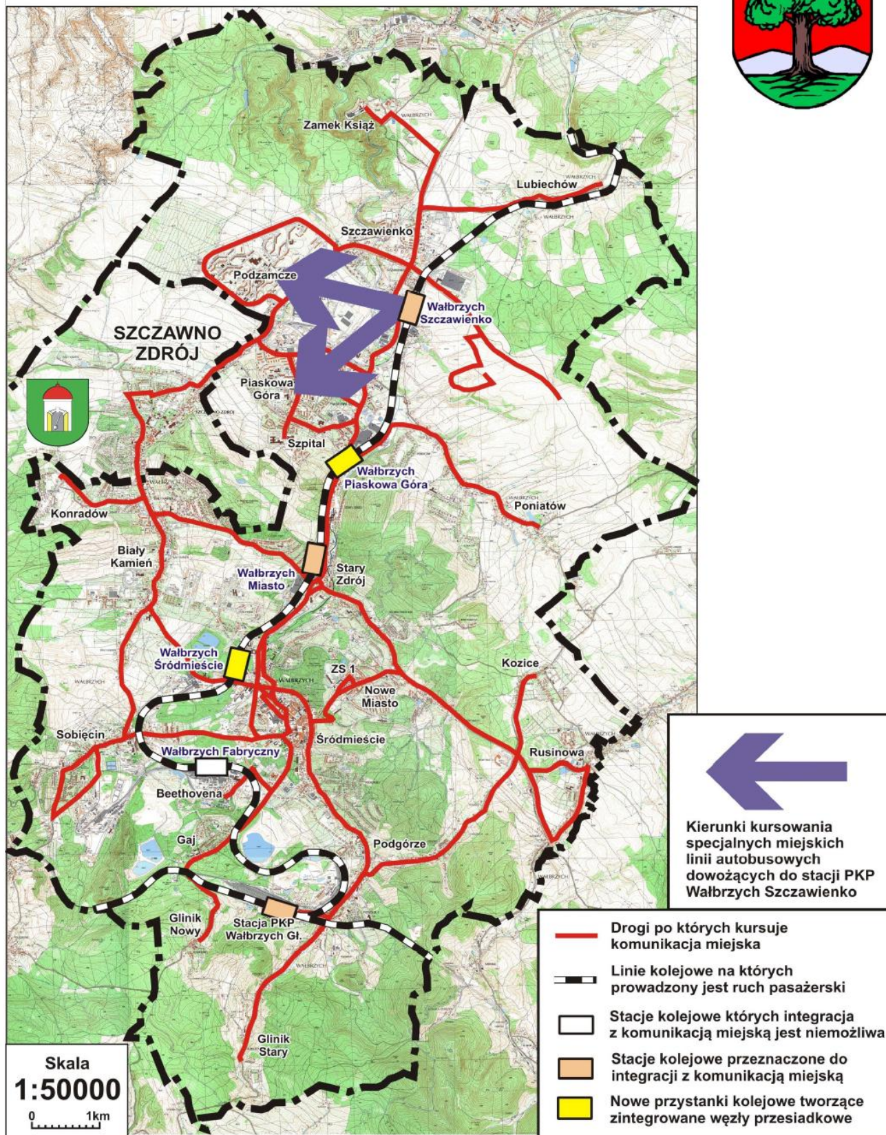
Rys. VIII.6. Integracja regionalnej komunikacji kolejowej z miejskim transportem publicznym na terenie Wałbrzysza.
