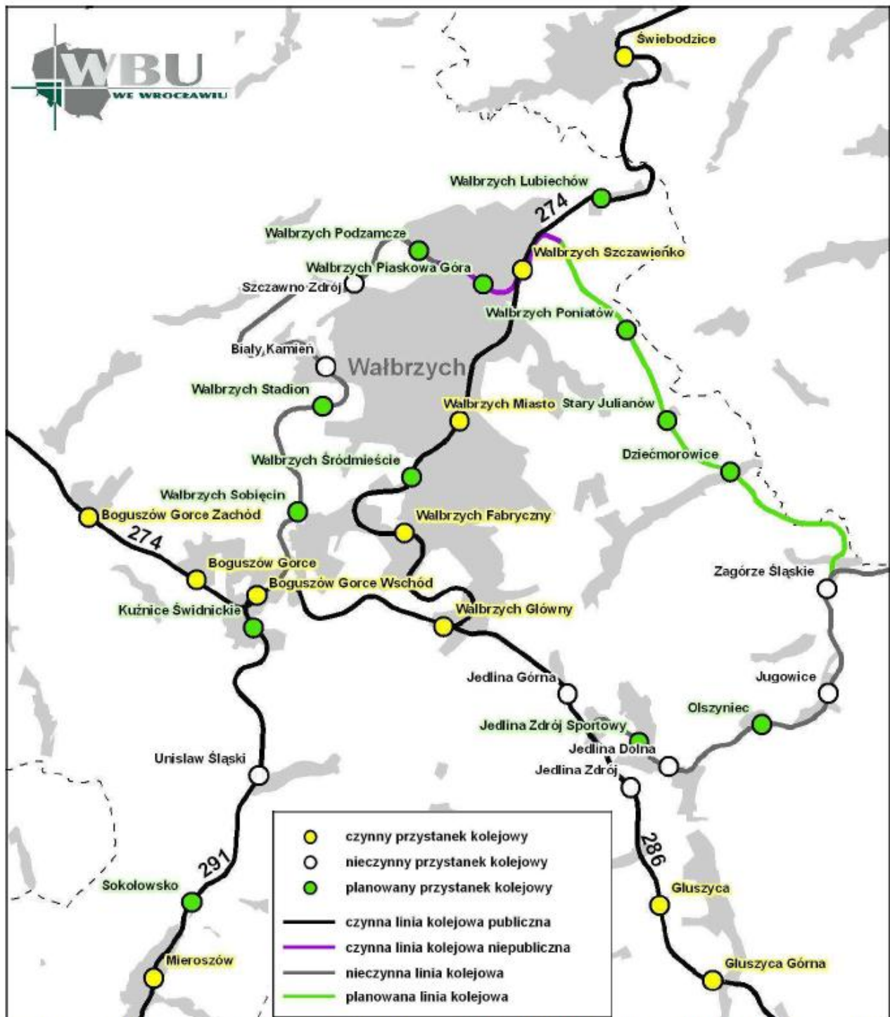
Rys. VIII.3. Siatka połączeń kolejowych powstałych w ramach Wałbrzyskiej Kolei Aglomeracyjnej wg koncepcji Wojewódzkiego Biura Urbanistycznego we Wrocławiu.
