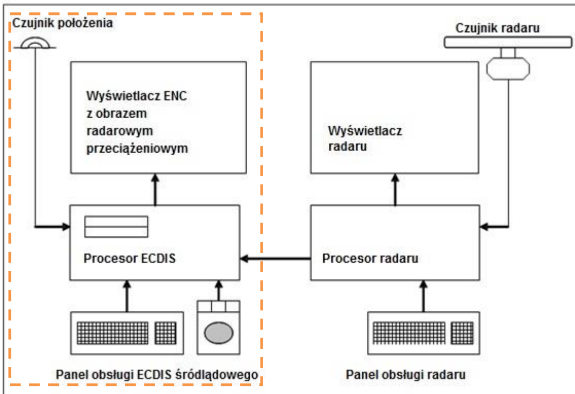
Rys. 1: Sprzęt ECDIS śródlądowy, niezależny sprzęt podłączony do sprzętu radarowego (konfiguracja systemu 2)
