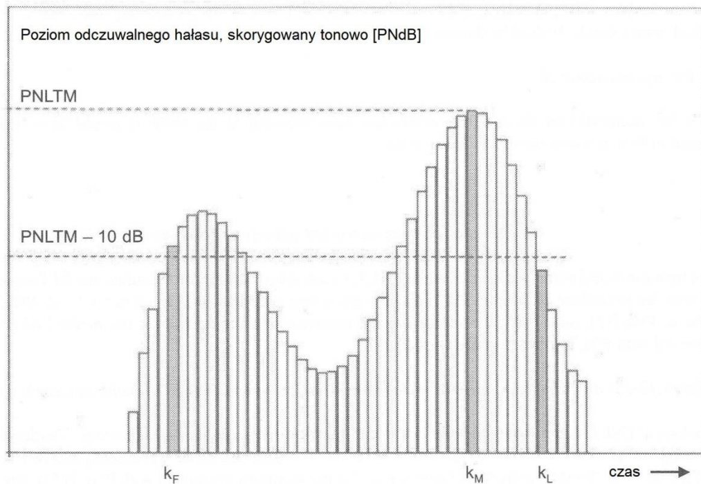
Rys. A2-2. Przykład przebiegu czasowego hałasu przelotu
