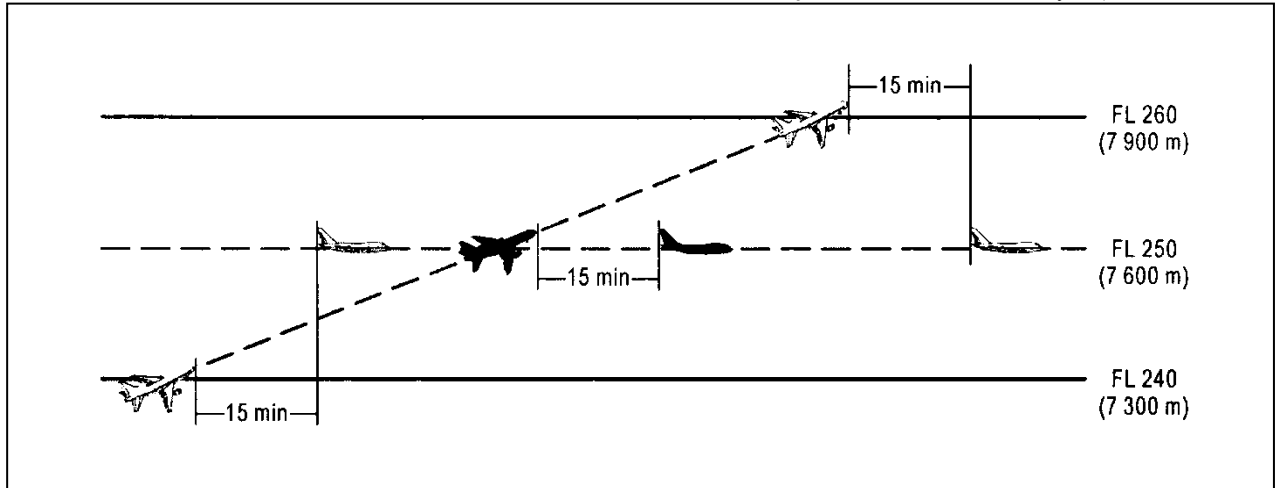
Rysunek 5-18A. Separacja piętnastominutowa między statkami powietrznymi podczas wznoszenia i na przecinających się liniach drogi (patrz pkt 5.4.2.2.2.2. lit. a))
