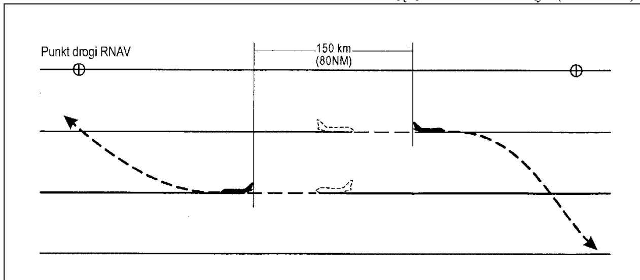
Rysunek 5-27. Separacja — przy stosowaniu RNAV — 150 km (80 NM) między statkami powietrznymi na przeciwnych liniach drogi (patrz pkt 5.4.2.5.7.)
