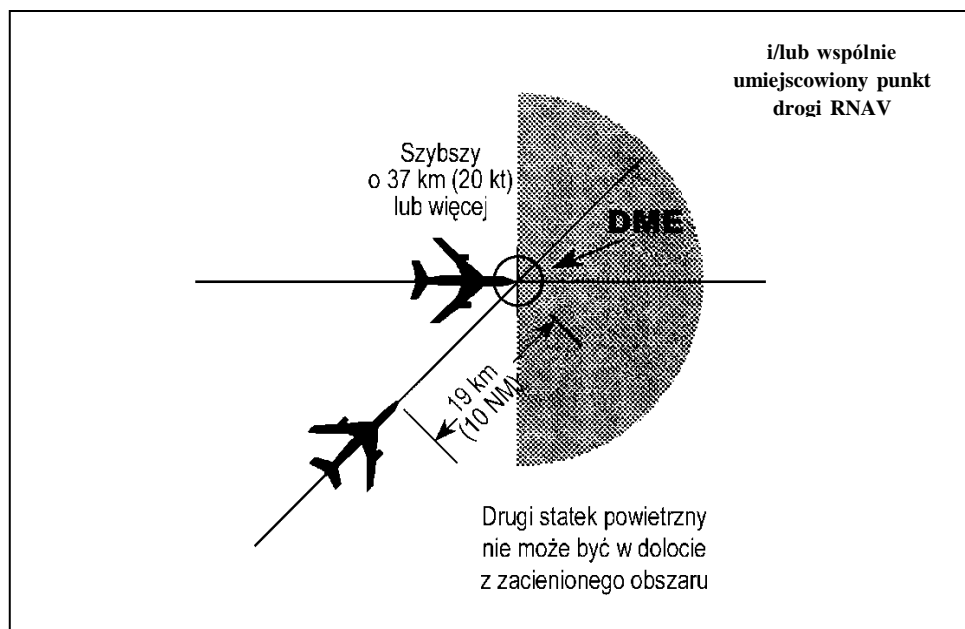
Rysunek 5-23B. Separacja — przy wykorzystaniu DME lub GNSS — 19 km (10 NM) między statkami powietrznymi na przecinających się liniach drogi i na tym samym poziomie lotu (patrz pkt 5.4.2.3.2.2.)
