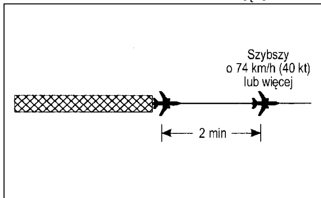
Rysunek 5-36. Separacja dwuminutowa między statkami powietrznymi lecącymi po tej samej linii drogi (patrz pkt 5.6.2.)
