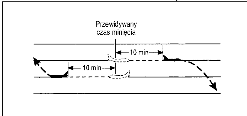
Rysunek 5-20. Separacja dziesięciominutowa między statkami powietrznymi na przecinających się liniach drogi (patrz pkt 5.4.2.2.3.)
