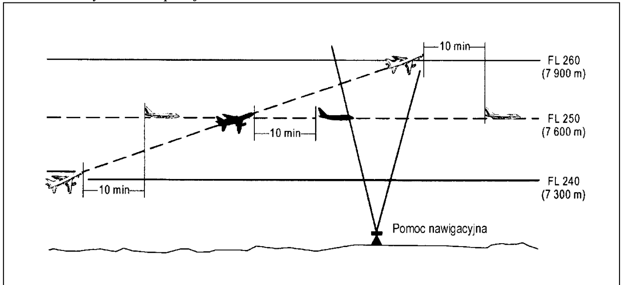
Rysunek 5-19A. Separacja dziesięciominutowa między statkami powietrznymi podczas wznoszenia i na przecinających się liniach drogi (patrz pkt 5.4.2.2.2.2. lit. b))
