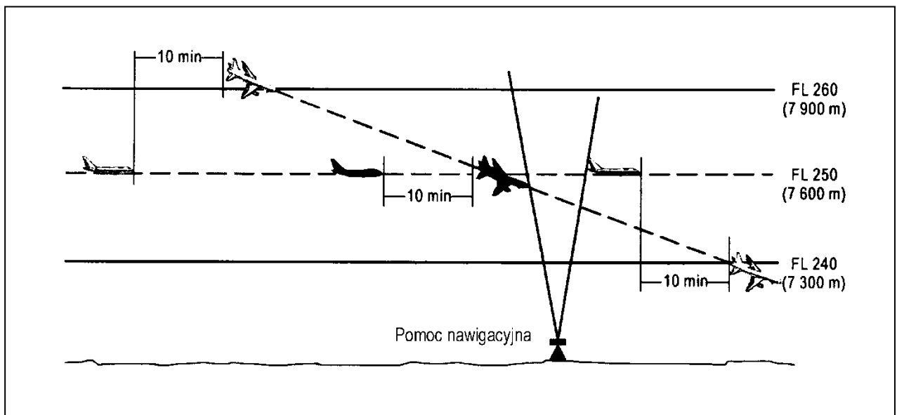
Rysunek 5-19B. Separacja dziesięciominutowa między statkami powietrznymi podczas zniżania i na przecinających się liniach drogi (patrz pkt 5.4.2.2.2.2. lit. b))
