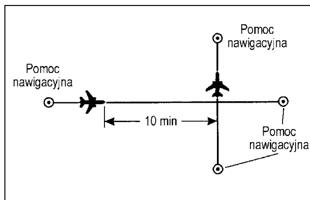
Rysunek 5-14. Separacja dziesięciominutowa między statkami powietrznymi na przecinających się liniach drogi i na tym samym poziomie lotu (patrz 5.4.2.2.1.2. b))
