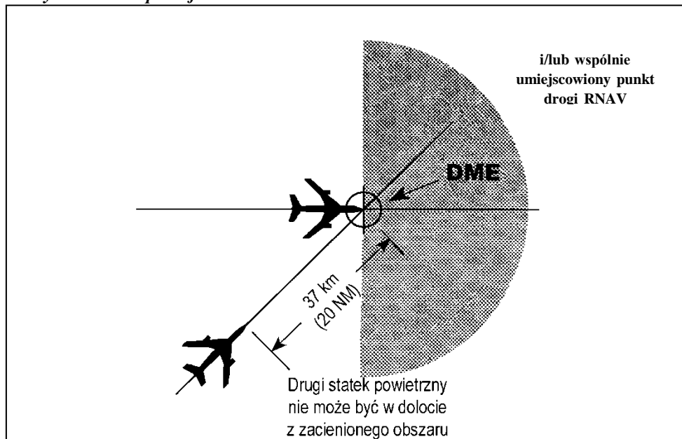
Rysunek 5-23A. Separacja — przy wykorzystaniu DME lub GNSS — 37 km (20 NM) między statkami powietrznymi na przecinających się liniach drogi i na tym samym poziomie lotu (patrz pkt 5.4.2.3.2.2.)
