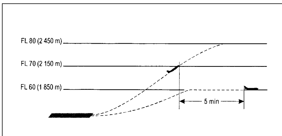
Rysunek 5-37. Separacja pięciominutowa między odlatującymi statkami powietrznymi lecącymi po tej samej linii drogi (patrz pkt 5.6.3.)
