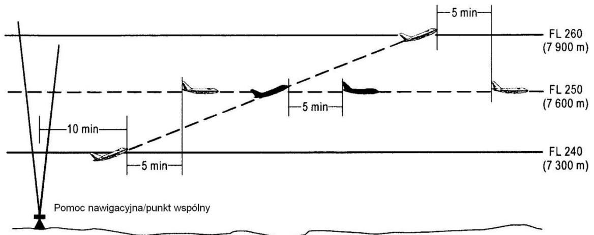
Rysunek 5-17A. Separacja pięciominutowa między statkami powietrznymi podczas wznoszenia i na tej samej linii drogi (patrz pkt 5.4.2.2.2.1. lit. c))
