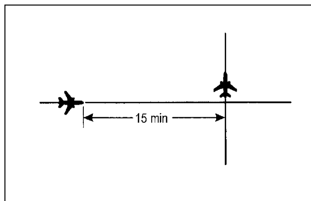
Rysunek 5-13. Separacja piętnastominutowa między statkami powietrznymi na przecinających się liniach drogi i na tym samym poziomie lotu (patrz pkt 5.4.2.2.1.2. lit a))
