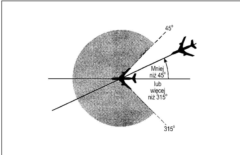
Rysunek 5-6. Statki powietrzne na tej samej linii drogi (patrz pkt 5.4.2.1.5. lit. a))
