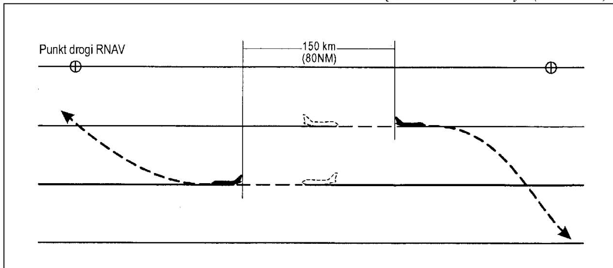
Rysunek 5-27. Separacja — przy stosowaniu RNAV — 150 km (80 NM) między statkami powietrznymi na przeciwnych trasach (patrz pkt 5.4.2.5.7.)
