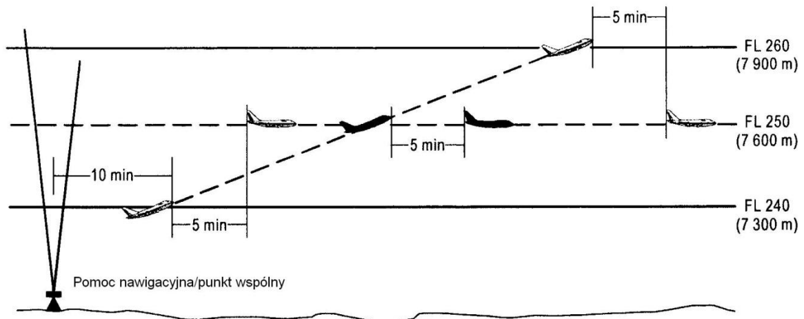
Rysunek 5-17A. Separacja pięciominutowa między statkami powietrznymi podczas wznoszenia i na tej samej linii drogi (patrz pkt 5.4.2.2.2.1. lit. c))
