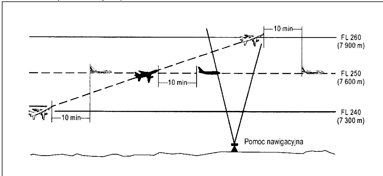
Rysunek 5-19A. Separacja dziesięciominutowa między statkami powietrznymi podczas wznoszenia i na przecinających się trakach (patrz pkt 5.4.2.2.2.2. lit. b))
