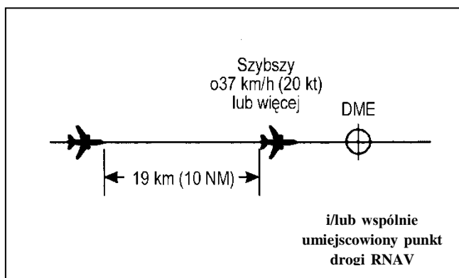
Rysunek 5-22. Separacja — przy wykorzystaniu DME lub GNSS — 19 km (10 NM) między statkami powietrznymi na tej samej linii drogi i na tym samym poziomie lotu (patrz pkt 5.4.2.3.2.1. lit. b))
