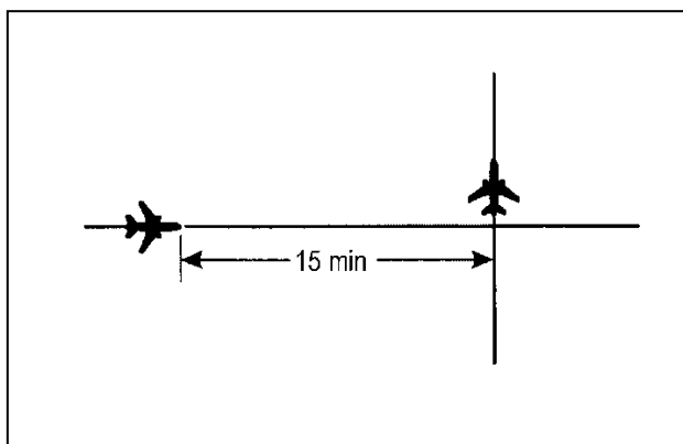
Rysunek 5-13. Separacja piętnastominutowa między statkami powietrznymi na przecinających się trackach i na tym samym poziomie lotu (patrz pkt 5.4.2.2.1.2. lit a))
