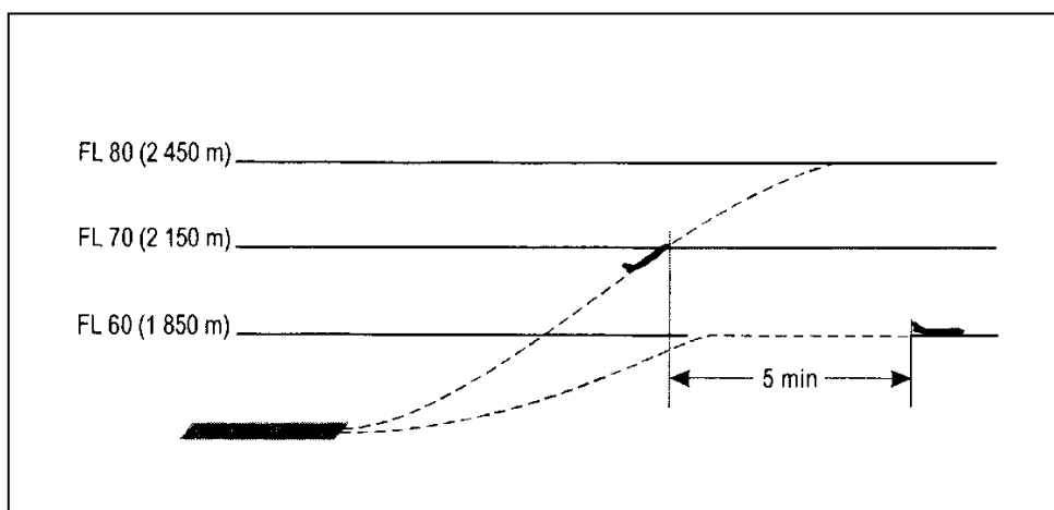
Rysunek 5-37. Separacja pięciominutowa między odlatującymi statkami powietrznymi lecącymi po tej samej linii drogi (patrz pkt 5.6.3.)
