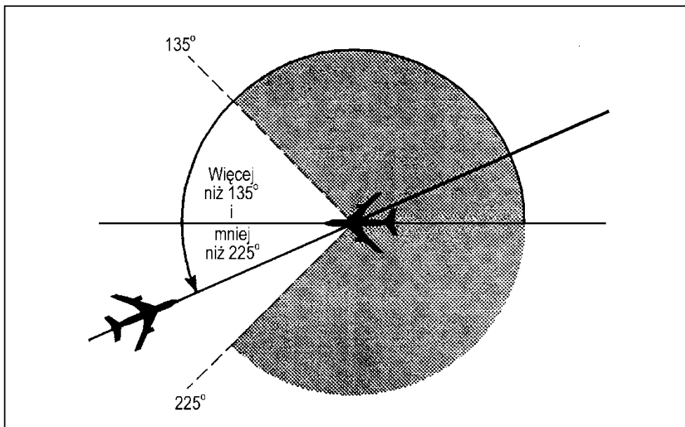
Rysunek 5-7. Statki powietrzne na traktach o przeciwnych kierunkach (patrz pkt 5.4.2. 1.5. lit. b))
