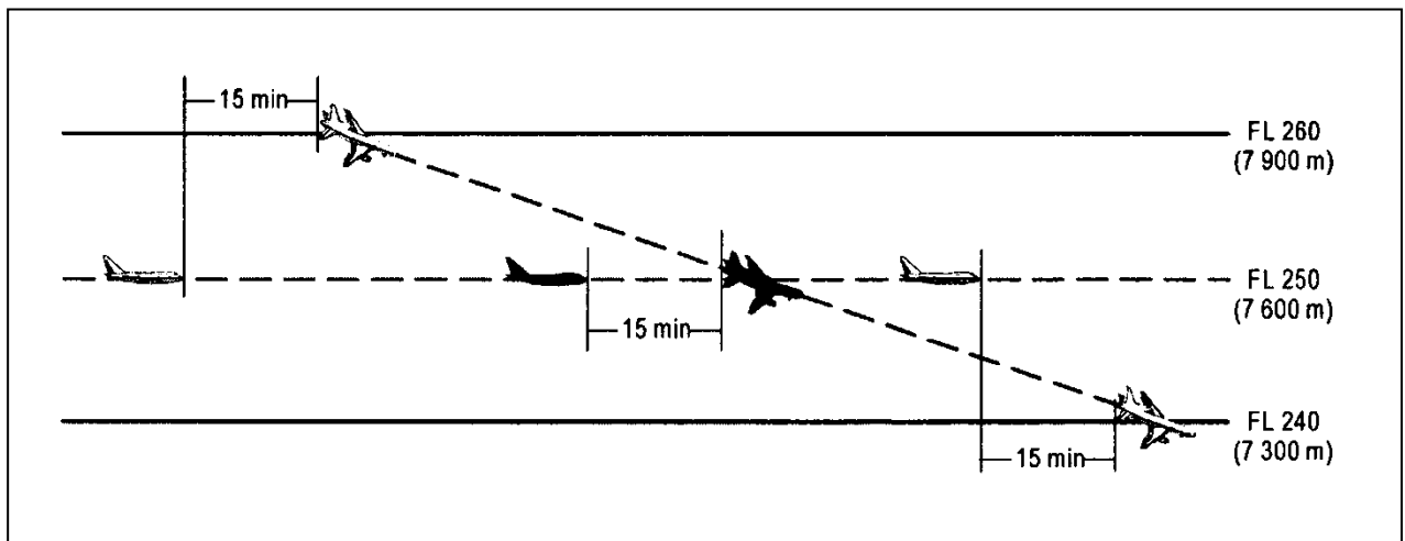
Rysunek 5-18B. Separacja piętnastominutowa między statkami powietrznymi podczas zniżania i na przecinających się trakach (patrz pkt 5.4.2.2.2.2. lit. a))
