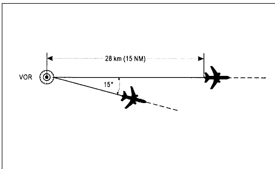
Rysunek 5-2. Separacja przy korzystaniu z tej samej pomocy nawigacyjnej — VOR (patrz pkt 5.4.1.2.1.2. a))
