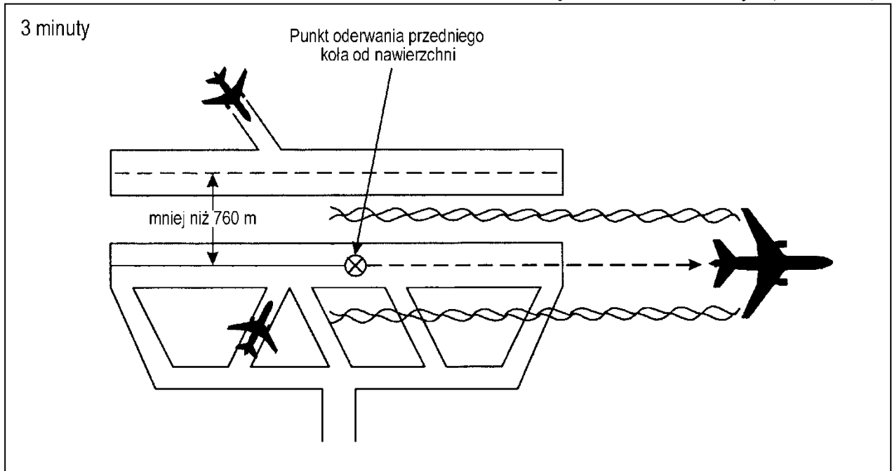
Rysunek 5-41. Separacja trzyminutowa między statkami powietrznymi lecącymi po tej samej linii drogi i która jest uwarunkowana turbulencją w śladzie aerodynamicznym (patrz pkt 5.8.3.2.)
