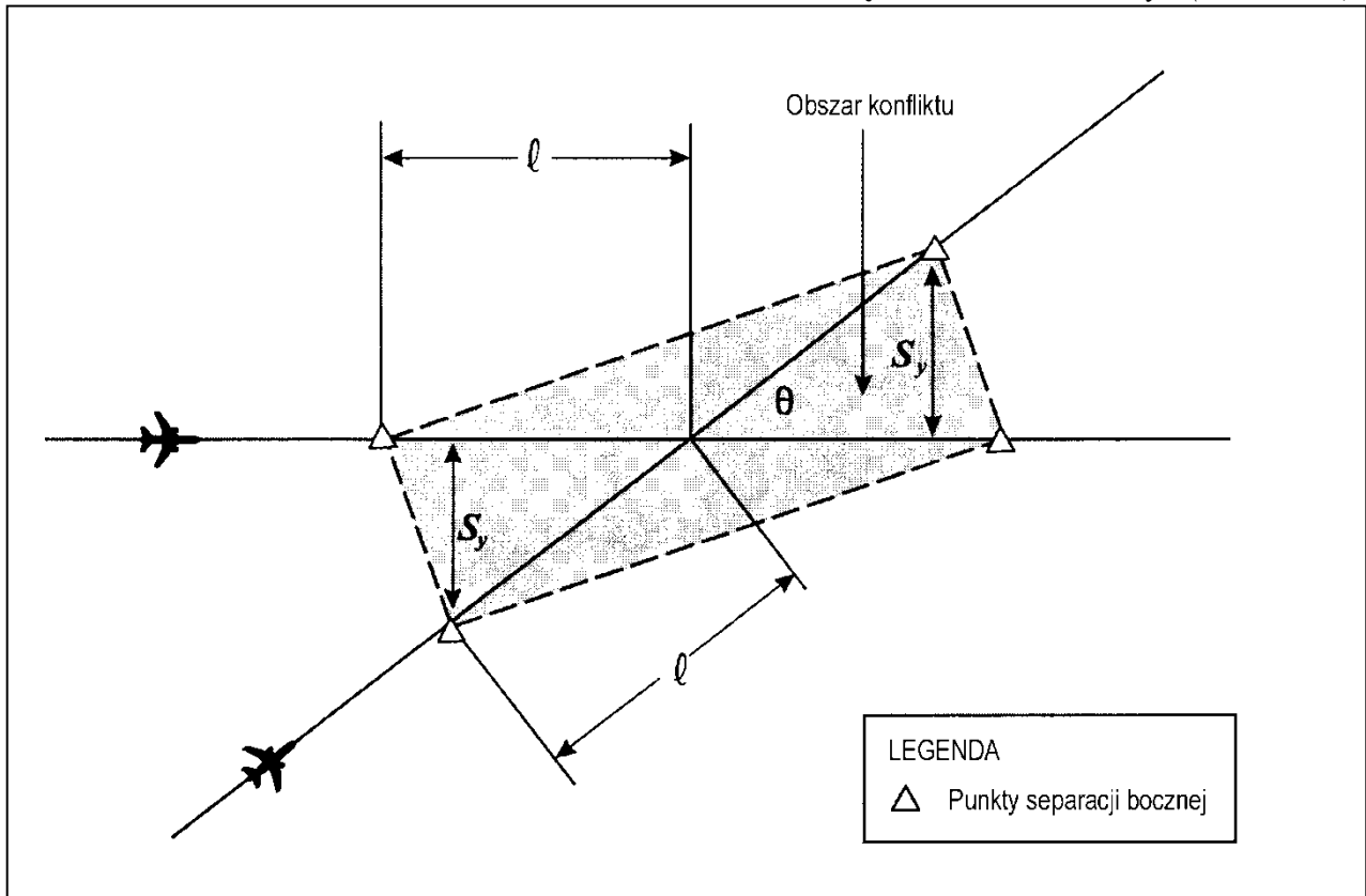
Rysunek 5-5. Punkty separacji bocznej i obszar konfliktu (patrz pkt 5.4.1.2.1.5.1.)
