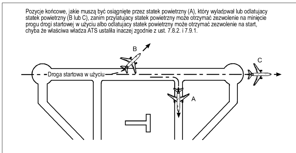
Rysunek 7- 3. Separacje między odlatującymi a przylatującymi statkami powietrznymi (patrz pkt 7.9.2. i 7.10.1.)
