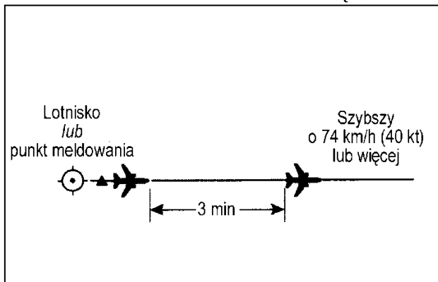
Rysunek 5-12. Separacja trzyminutowa między statkami powietrznymi na tej samej linii drogi i na tym samym poziomie lotu (patrz pkt 5.4.2.2.1.1. lit. d))
