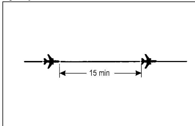
Rysunek 5-9. Separacja piętnastominutowa między statkami powietrznymi na tej samej linii drogi i na tym samym poziomie lotu (patrz pkt 5.4.2.2.1.1. lit. a))
