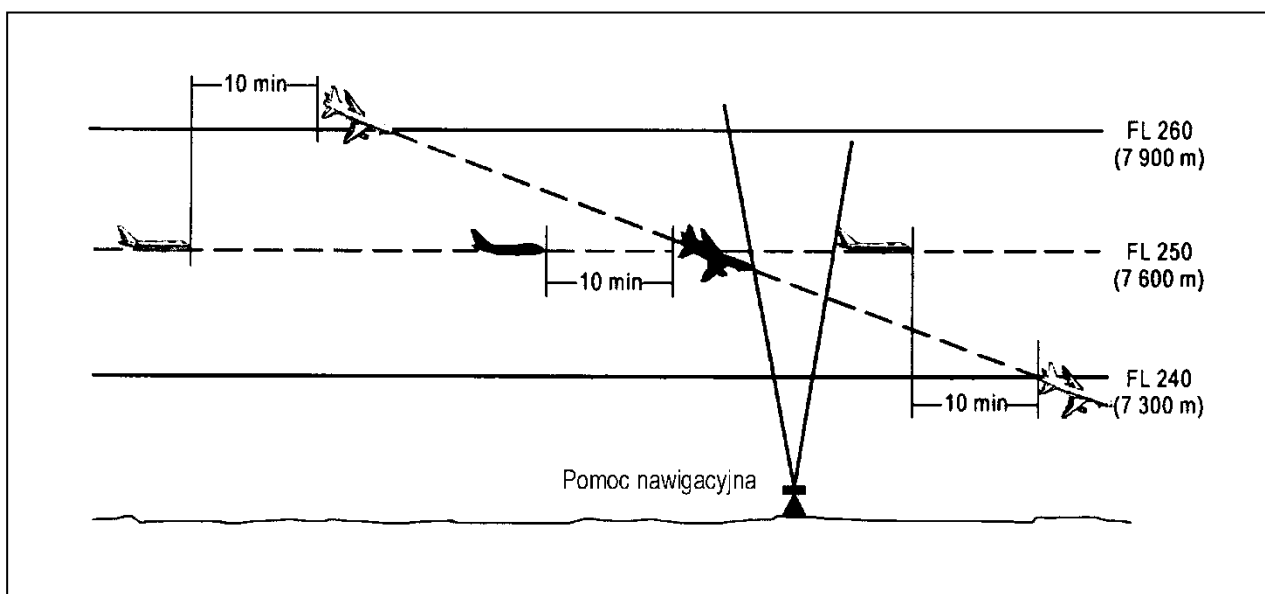
Rysunek 5-19B. Separacja dziesięciominutowa między statkami powietrznymi podczas zniżania i na przecinających się trakach (patrz pkt 5.4.2.2.2.2. lit. b))
