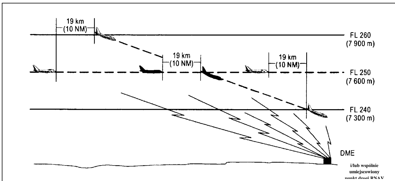
Rysunek 5-24B. Separacja — przy wykorzystaniu DME lub GNSS — 19 km (10 NM) między statkami powietrznymi podczas zniżania na tej samej linii drogi (patrz pkt 5.4.2.3.2.3. lit. c))
