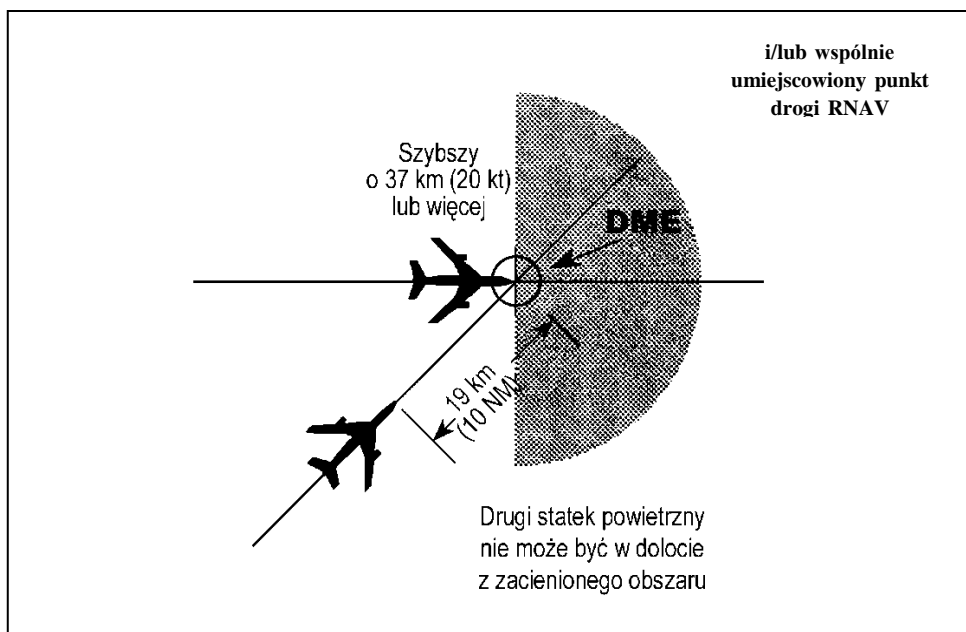
Rysunek 5-23B. Separacja — przy wykorzystaniu DME lub GNSS — 19 km (10 NM) między statkami powietrznymi na przecinających się trakach i na tym samym poziomie lotu (patrz pkt 5.4.2.3.2.2.)
