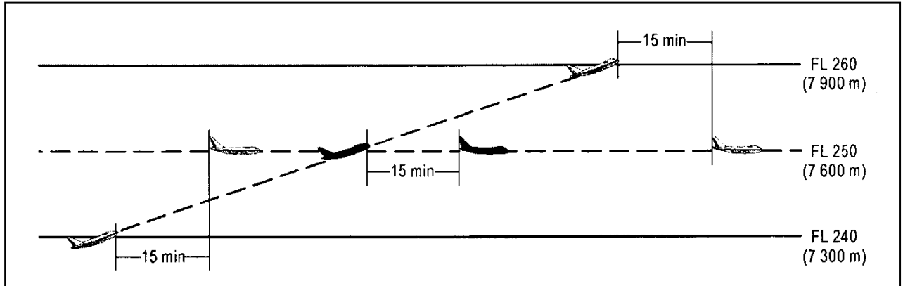
Rysunek 5-15A. Separacja piętnastominutowa między statkami powietrznymi podczas wznoszenia i na tej samej linii drogi (patrz pkt 5.4.2.2.2.1. lit. a))
