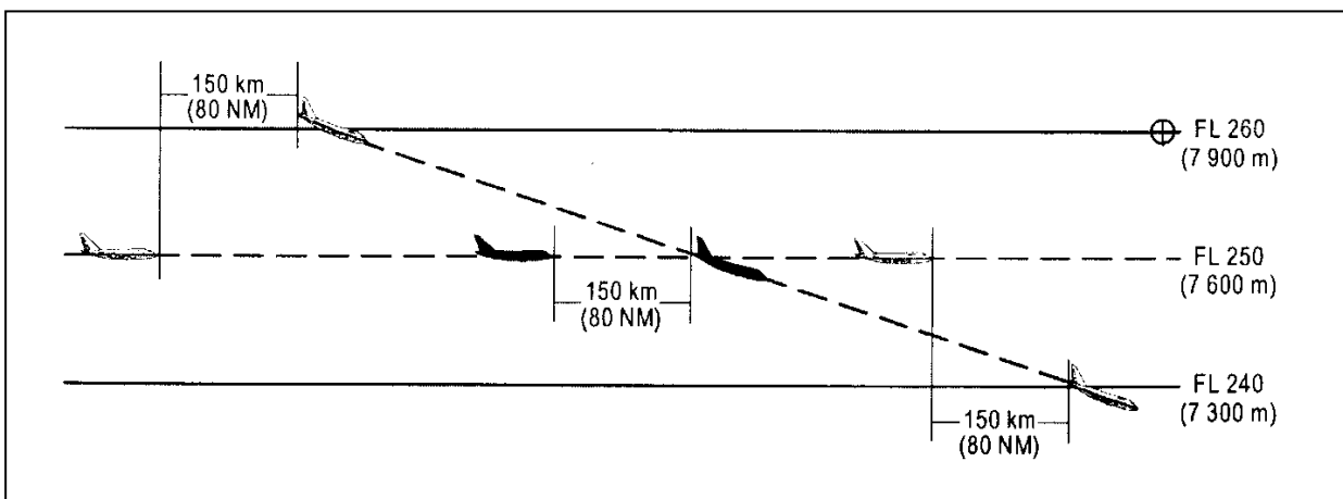
Rysunek 5-26B. Separacja — przy stosowaniu RNAV — 150 km (80 NM) między statkami powietrznymi podczas zniżania na tej samej linii drogi (patrz pkt 5.4.2.5.5. lit. e))
