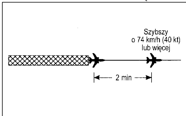
Rysunek 5-36. Separacja dwuminutowa między statkami powietrznymi lecącymi po tej samej linii drogi (patrz pkt 5.6.2.)
