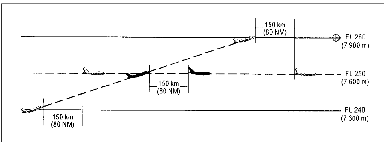
Rysunek 5-26A. Separacja — przy stosowaniu RNAV — 150 km (80 NM) między statkami powietrznymi podczas wznoszenia na tej samej linii drogi (patrz pkt 5.4.2.5.5. lit. c))
