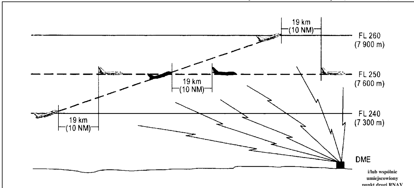
Rysunek 5-24A. Separacja — przy wykorzystaniu DME lub GNSS — 19 km (10 NM) podczas wznoszenia na tej samej linii drogi (patrz pkt 5.4.2.3.2.3. lit. c))
