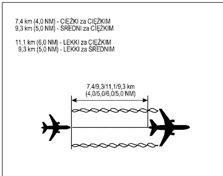
Rysunek 8-1A. Statek powietrzny wykonuje lot bezpośredni za poprzedzającym statkiem powietrznym (patrz pkt 8.7.3.4 i 8.7.3.4.1)
