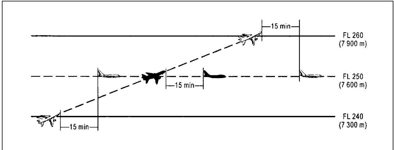
Rysunek 5-18A. Separacja piętnastominutowa między statkami powietrznymi podczas wznoszenia i na przecinających się trakach (patrz pkt 5.4.2.2.2.2. lit. a))
