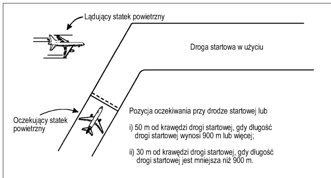
Rysunek 7-2. Pozycja oczekiwania dla statków powietrznych (patrz pkt 7.5.3.1.3.2.)
