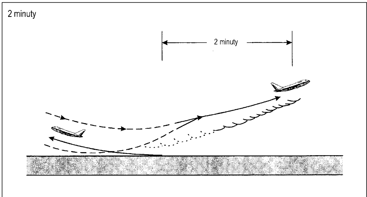
Rysunek 5-42. Separacja dwuminutowa między statkami powietrznymi startującymi w przeciwnych kierunkach i która jest uwarunkowana turbulencją w śladzie aerodynamicznym (patrz pkt 5.8.5. lit. a))
