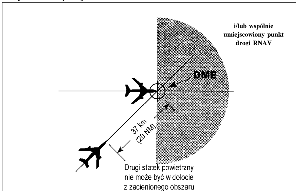
Rysunek 5-23A. Separacja — przy wykorzystaniu DME lub GNSS — 37 km (20 NM) między statkami powietrznymi na przecinających się trakach i na tym samym poziomie lotu (patrz pkt 5.4.2.3.2.2.)
