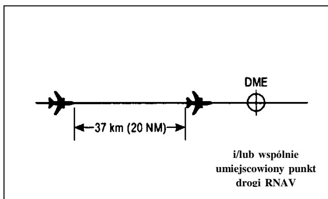
Rysunek 5-21. Separacja — przy wykorzystaniu DME lub GNSS — 37 km (20 NM) między statkami powietrznymi na tej samej linii drogi i na tym samym poziomie lotu (patrz pkt 5.4.2.3.2.1. lit. a))
