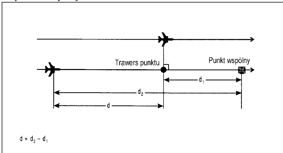
Rysunek 5-33. Obliczanie odległości podłużnej między statkami powietrznymi — równoległe linie drogi (patrz pkt 5.4.2.6.4.1. lit. c)
