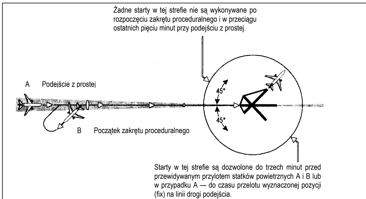
Rysunek 5-37. Separacja pięciominutowa między odlatującymi statkami powietrznymi lecącymi po tej samej linii drogi (patrz pkt 5.6.3.)
