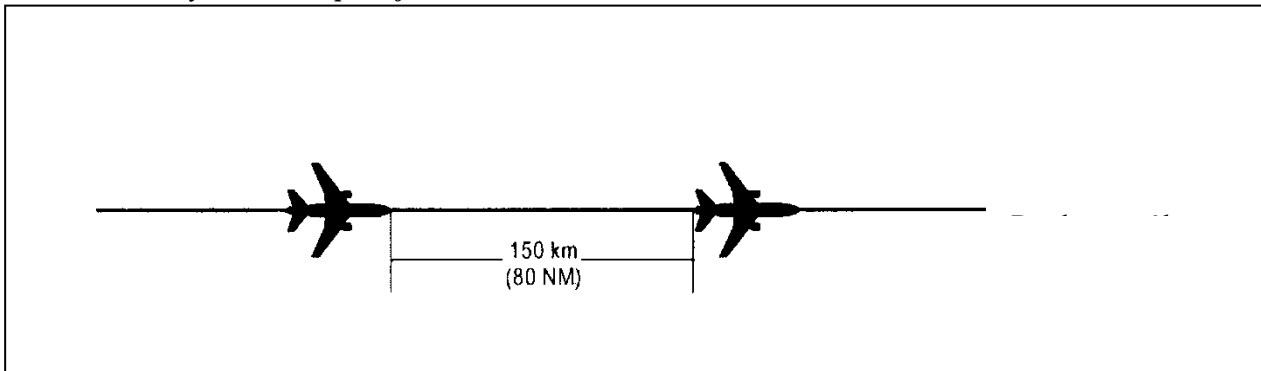
Rysunek 5-25. Separacja — przy stosowaniu RNAV — 150 km (80 NM) między statkami powietrznymi na tym samym poziomie lotu (patrz pkt 5.4.2.5.5. lit. b))
