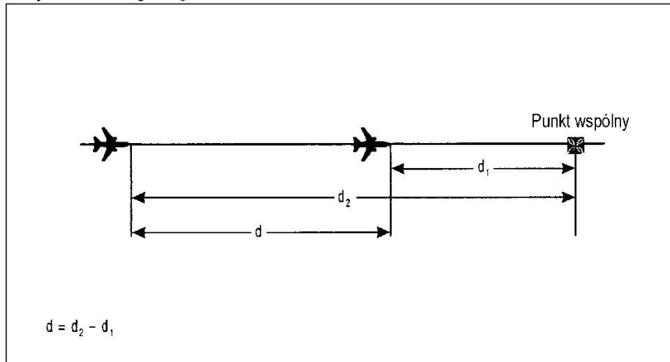
Rysunek 5-28. Obliczanie odległości podłużnej między statkami powietrznymi — identyczna linia drogi, ten sam kierunek (patrz pkt 5.4.2.6.4.1. lit. a))
