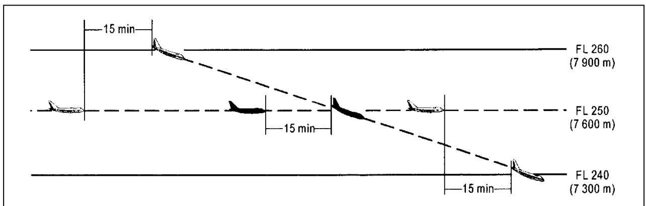
Rysunek 5-15B. Separacja piętnastominutowa między statkami powietrznymi podczas zniżania i na tej samej linii drogi (patrz pkt 5.4.2.2.2.1. lit. a))
