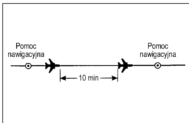
Rysunek 5-10. Separacja dziesięciminutowa między statkami powietrznymi na tej samej linii drogi i na tym samym poziomie lotu (patrz pkt 5.4.2.2.1.1. lit. b))
