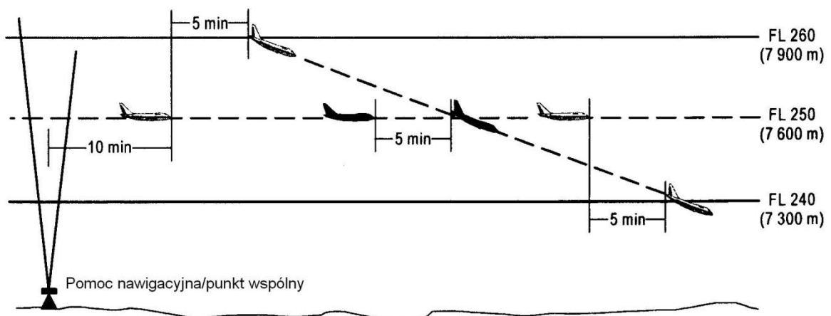
Rysunek 5-17B. Separacja pięciominutowa między statkami powietrznymi podczas zniżania i na tej samej linii drogi (patrz pkt 5.4.2.2.2.1. lit. c))
