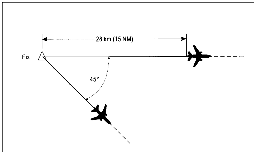
Rysunek 5-4. Separacja przy zastosowaniu metody zliczania drogi (patrz pkt 5.4.1.2.1.2. lit. c))
