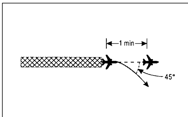
Rysunek 5-35. Separacja jednoczynowa między odlatającymi statkami powietrznymi z kątami drogi różniącymi się nie mniej niż 45° (patrz pkt 5.6.1.)
