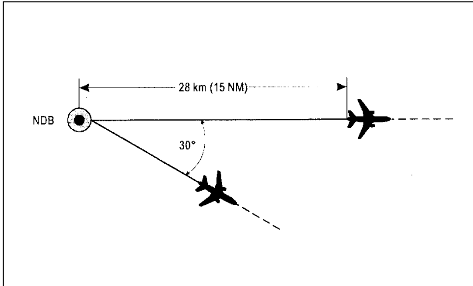
Rysunek 5-3. Separacja przy korzystaniu z tej samej pomocy nawigacyjnej — NDB (patrz pkt 5.4.1.2.1.2. lit. b))
