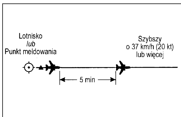
Rysunek 5-11. Separacja pięciminutowa między statkami powietrznymi na tej samej linii drogi i na tym samym poziomie lotu (patrz pkt 5.4.2.2.1.1. lit. c))
