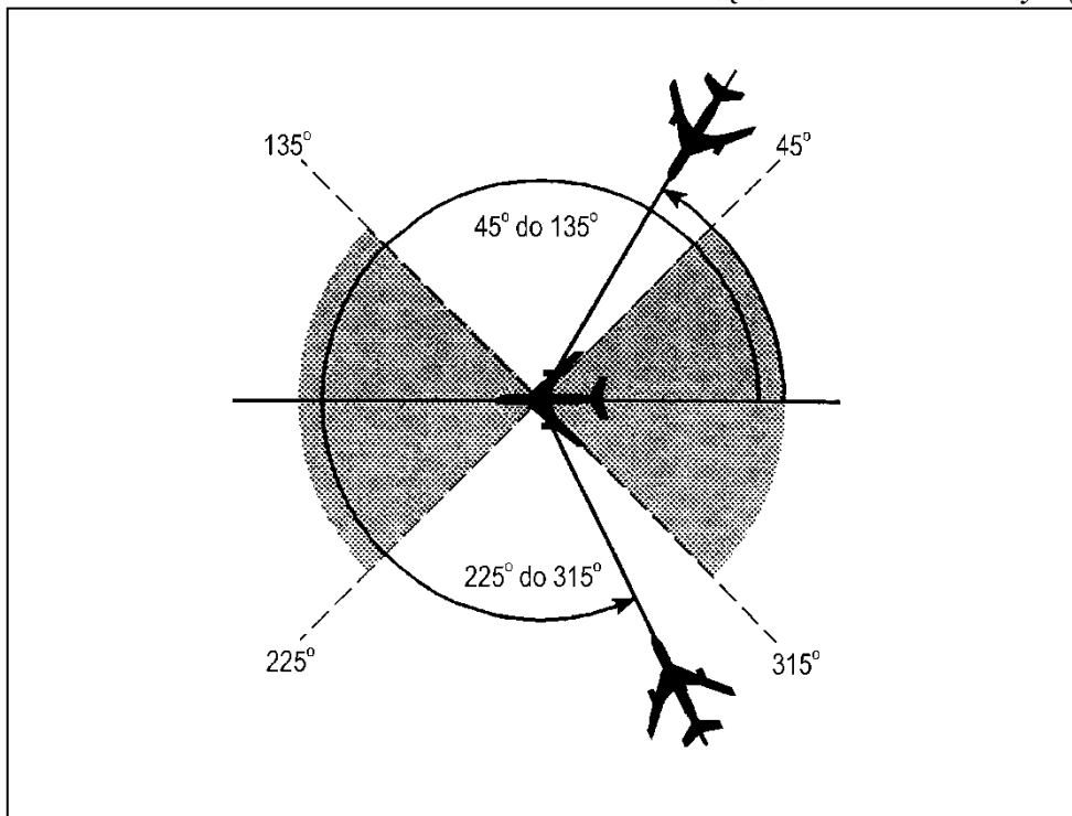
Rysunek 5-8. Statki powietrzne na przecinających się trackach (patrz pkt 5.4.2.1.5. lit. c))
