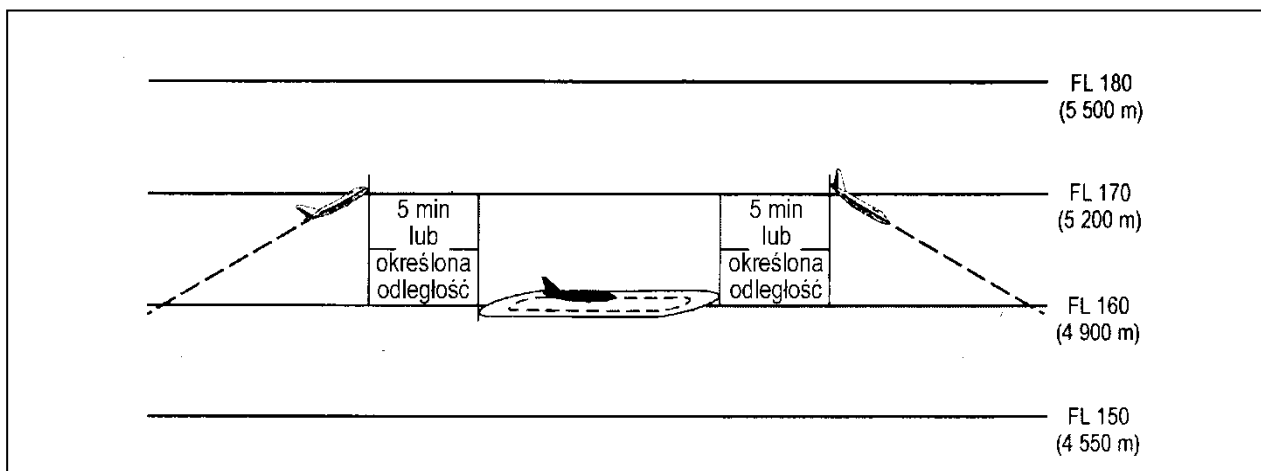
Rysunek 5-34. Separacja między statkami powietrznymi w oczekiwaniu a statkami powietrznymi na trasie (patrz pkt 5.5.2.)
