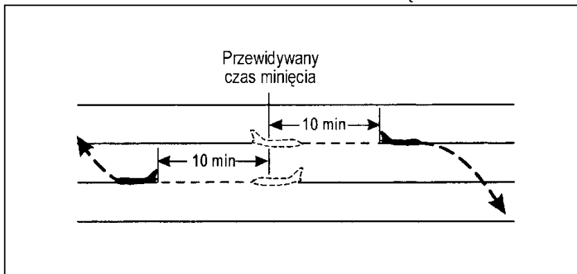
Rysunek 5-20. Separacja dziesięciominutowa między statkami powietrznymi na przecinających się trakach (patrz pkt 5.4.2.2.3.)
