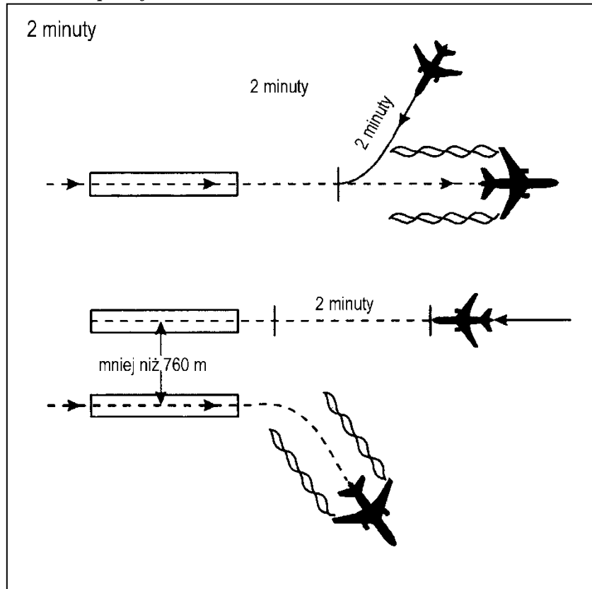
Rysunek 5-43. Separacja dwuminutowa między statkami powietrznymi przy lądowaniu z przeciwnego kierunku i która jest uwarunkowana turbulencją w śladzie aerodynamicznym (patrz pkt 5.8.5. lit. b))
