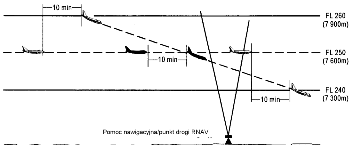
Rysunek 5-16B. Separacja dziesięciominutowa między statkami powietrznymi podczas zniżania i na tej samej linii drogi (patrz pkt 5.4.2.2.2.1. lit. b))
