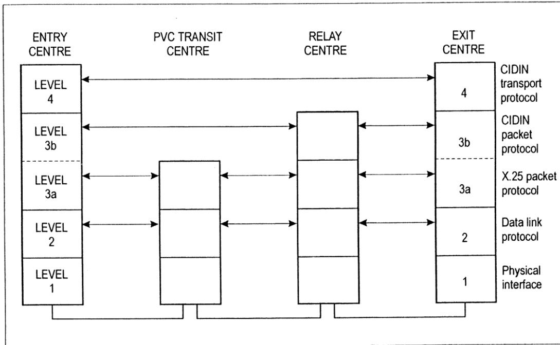
Rysunek 8-1. Poziomy protokół CIDIN
