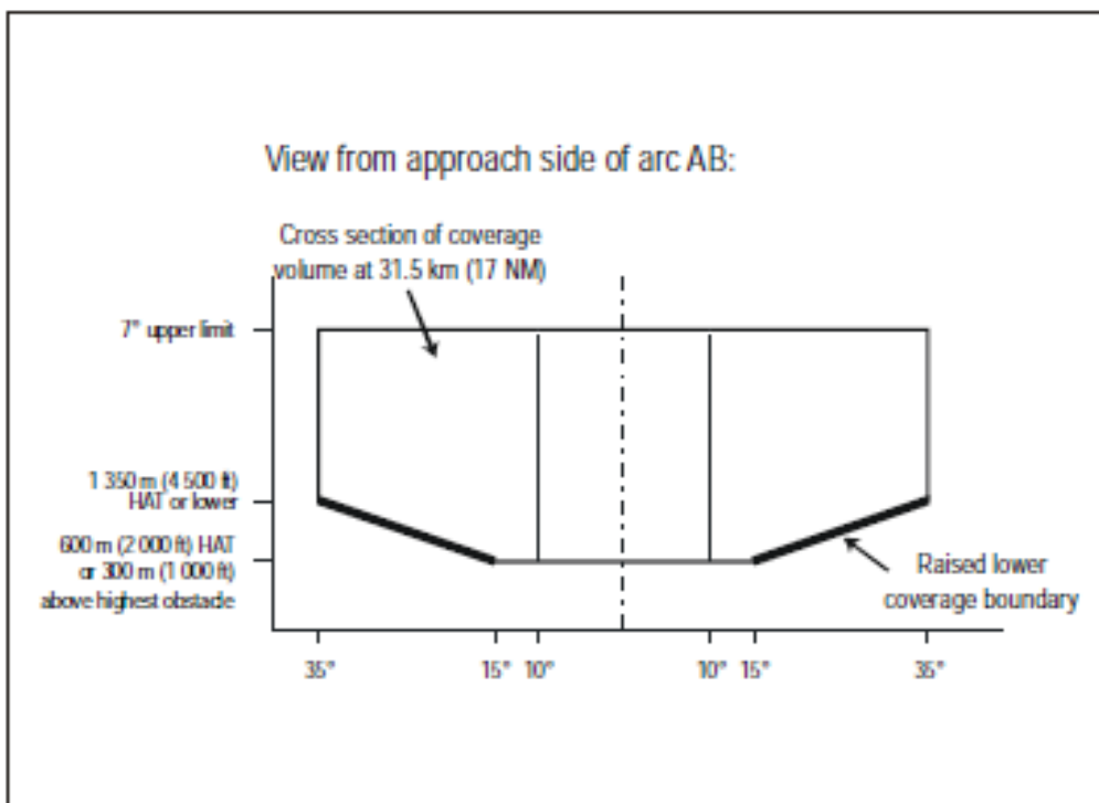
Rysunek C-8A. Pokrycie radiolatarni kierunku względem ewalacji
