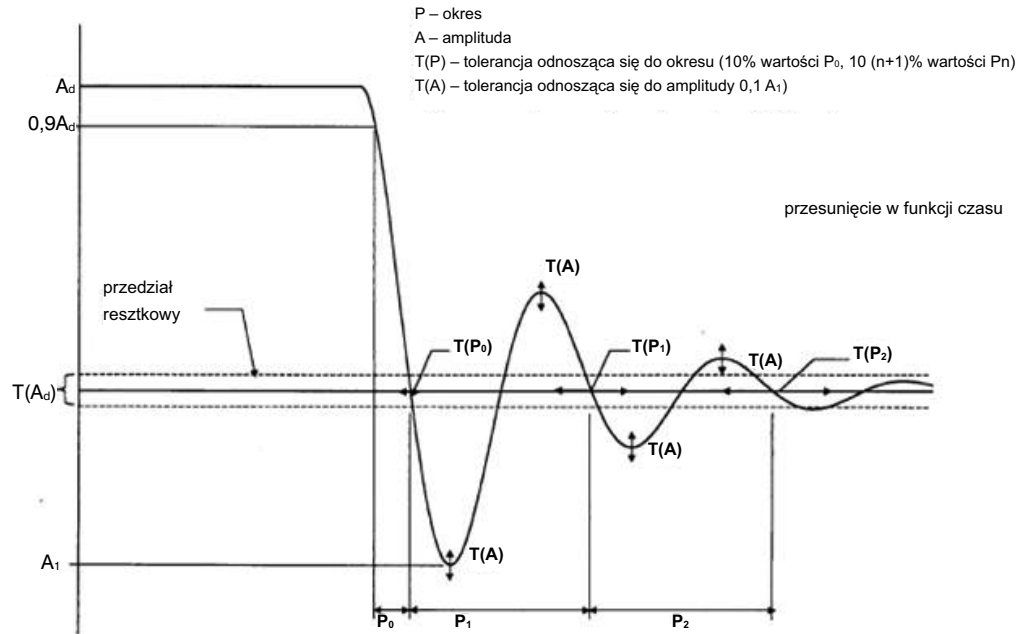
Rys. 1 Niedotłumiona odpowiedź na pobudzenie stopniowane
