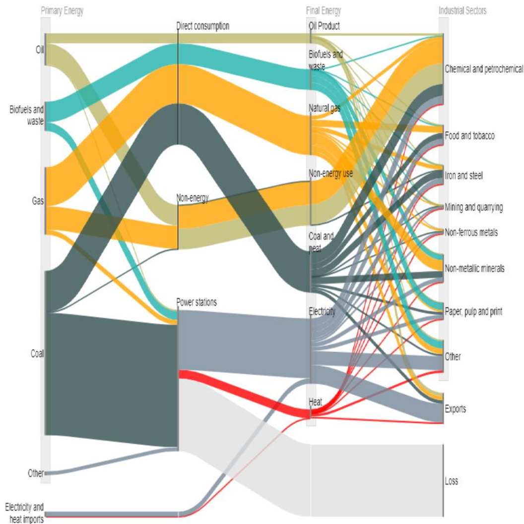
Rys. 1. Wykorzystanie energii przemysłowej w Polsce (2015), śledzone z energii pierwotnej do finalnej (w petadżulach, PJ)
