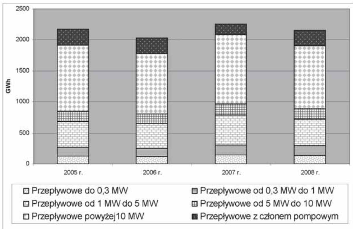
Rysunek 4 — Produkcja energii elektrycznej w elektrowniach wodnych w latach 2005–2008 w Polsce
