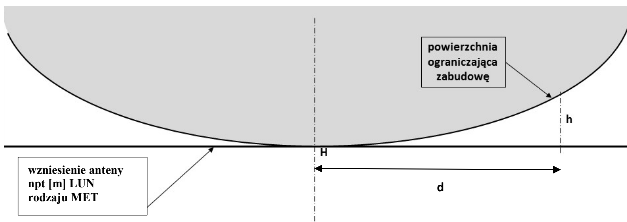
Rys. 5. 40) Kształt i wymiary powierzchni ograniczających zabudowę wokół dookólnych lotniczych urządzeń naziemnych rodzaju MET przeznaczonych do obserwacji meteorologicznych
