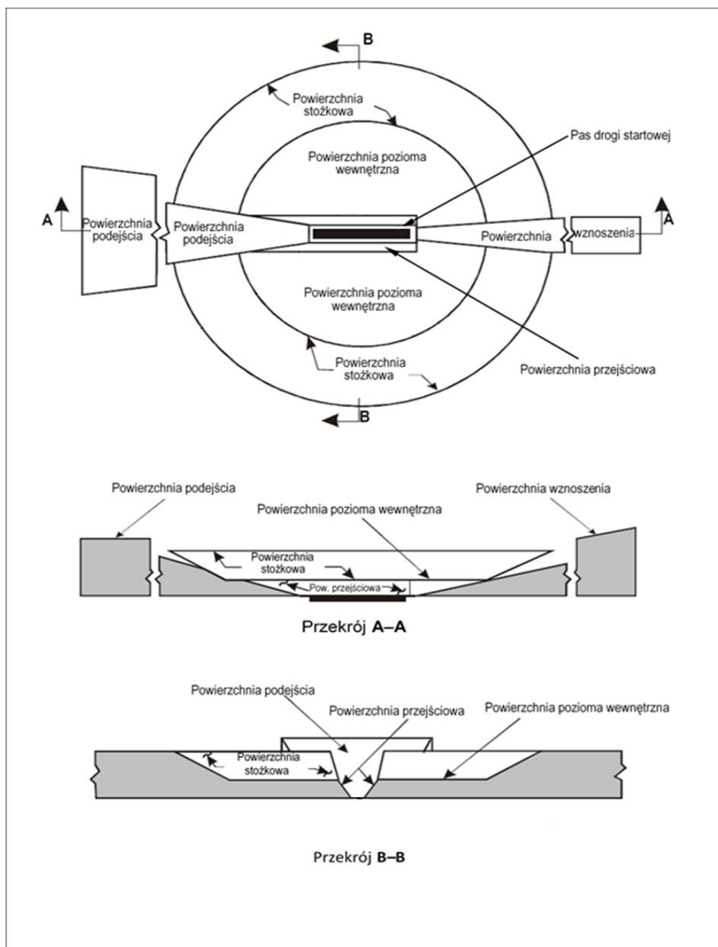
Rysunek 1. Schemat wyznaczania powierzchni stożkowej, powierzchni poziomej wewnętrznej, powierzchni podejścia, powierzchni przejściowej i powierzchni wznoszenia dla dróg startowych na lotniskach dla samolotów
