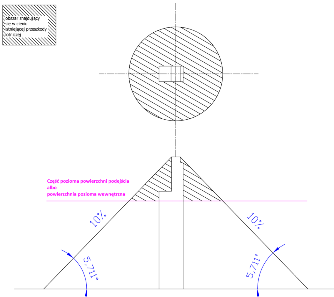
Rysunek 2. Schemat wyznaczania obszaru znajdującego się w cieniu istniejącej przeszkody lotniczej w części poziomej powierzchni podejścia, powierzchni stożkowej albo powierzchni poziomej wewnętrznej
