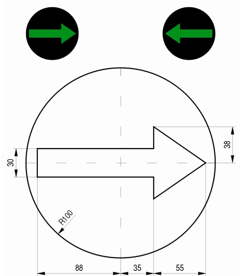
Rys. 10.10. Strzałka dopuszczająca skręcenie we wskazanym kierunku w prawo lub w lewo (odbicie zwierciadlane)
