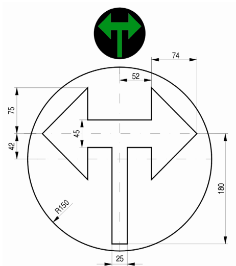
Rys. 10.7. Strzałki kierunku jazdy w prawo i w lewo dla sygnału zielonego
