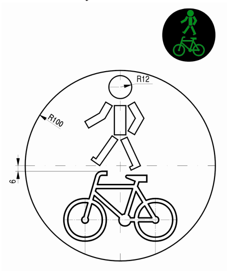
Rys. 10.22. Sylwetki pieszego i rowerzysty wspólnie w sygnale zielonym; szablon pieszego według konstrukcji na rys. 10.19 należy zmniejszyć o 40%, a szablon roweru według konstrukcji na rys. 10.21 – o 30%
