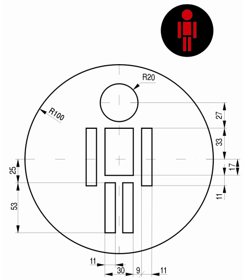
Rys. 10.20. Sylwetka pieszego w sygnale czerwonym dla pieszych
