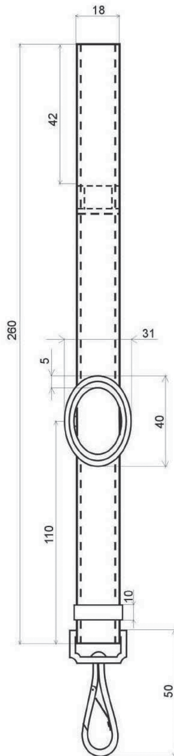
WYMIARY widok z przodu
