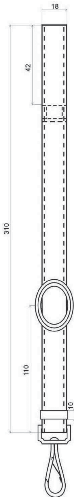
WYMIARY widok z przodu
