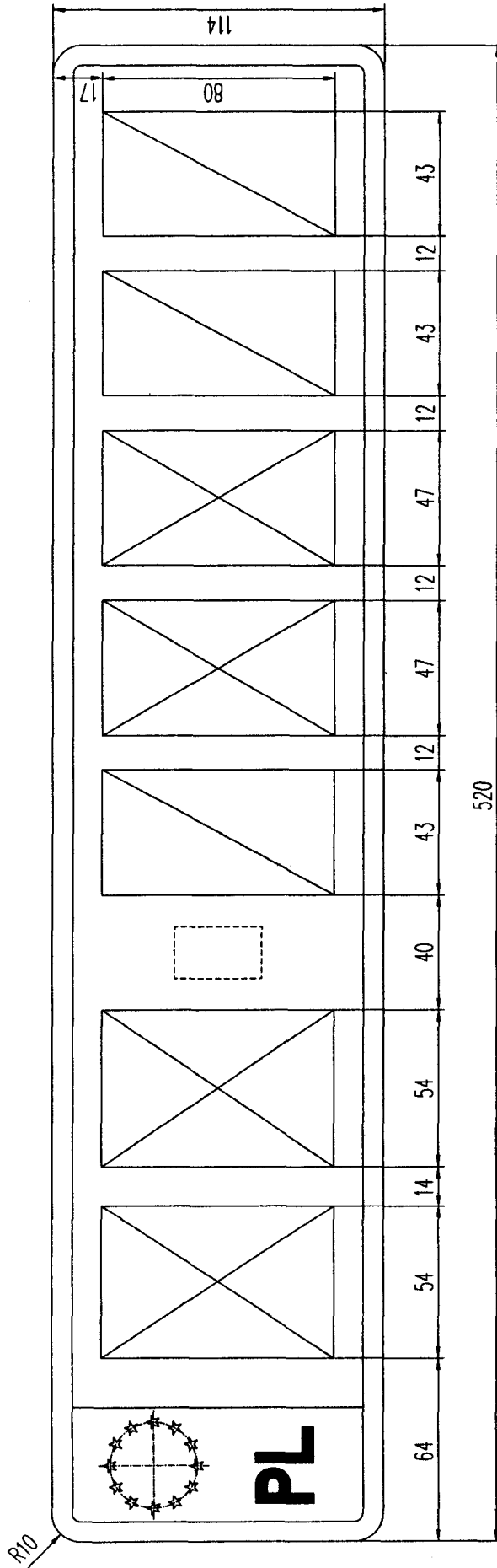
Rysunek 13b. Tablica samochodowa zwyczajna jednorzędowa (2 litery, 1 cyfra, 2 litery, 2 cyfry)
