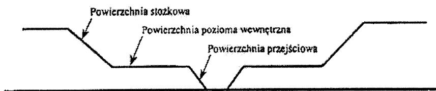
PRZEKRÓJ B-B
