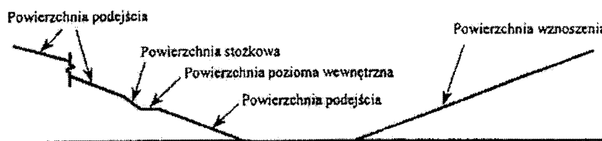
PRZEKRÓJ A-A
