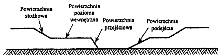
PRZEKRÓJ A-A
